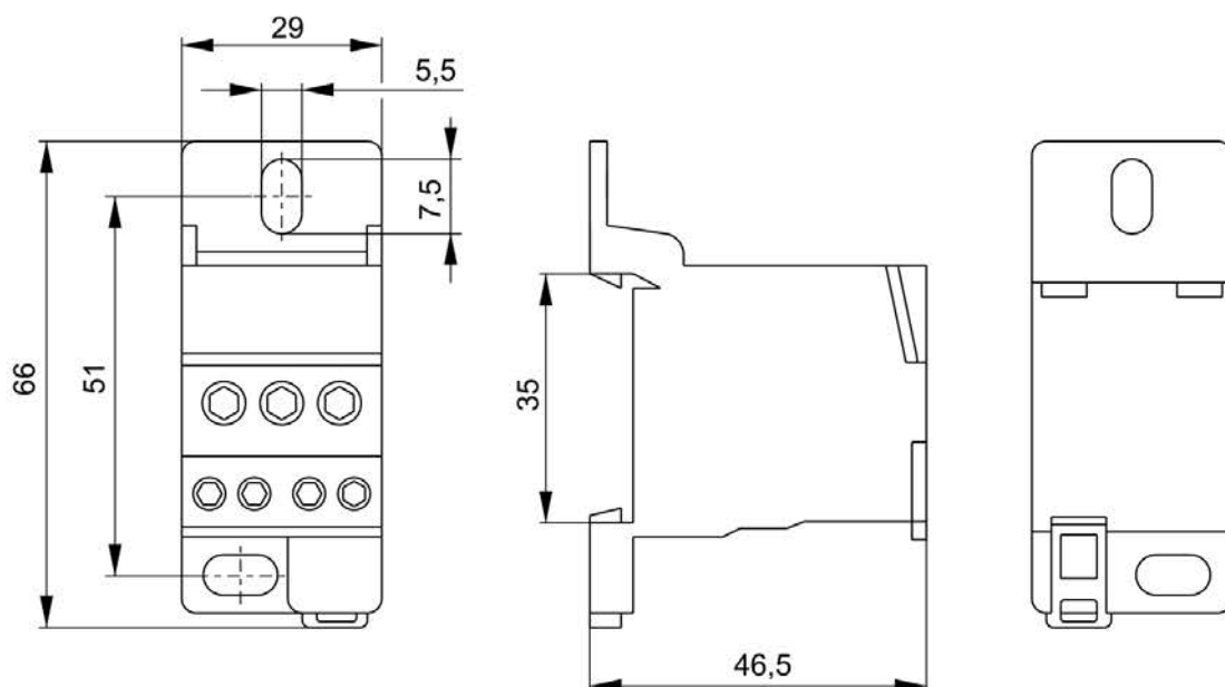
Рисунок 1 – Блоки распределительные РБД-80А
