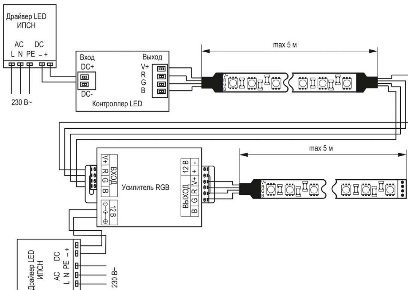
Рисунок 10 – Схема последовательного подключения RGB-усилителя
