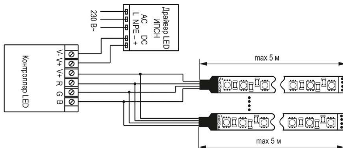
Рисунок 8 – Схема параллельного подключения многоцветной RGB светодиодной ленты к блоку питания и контроллеру
