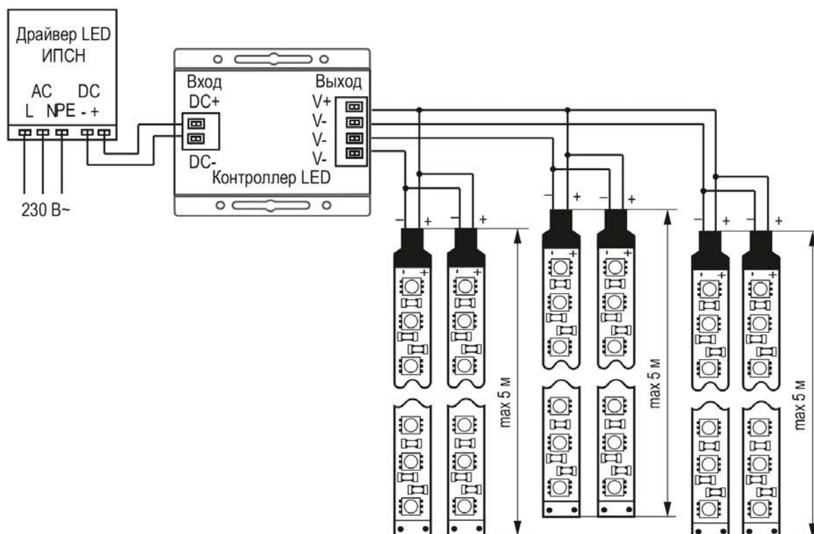
Рисунок 6 – Схема параллельного подключения одноцветных лент разного цвета к отдельному каналу контроллера с общим анодом
