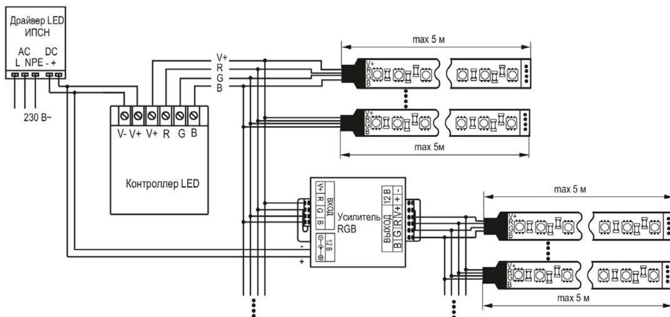
Рисунок 11 – Схема параллельного подключения RGB-усилителя
