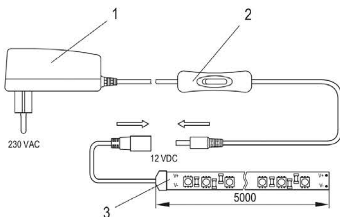
Рисунок 13 – Подключение LSR1-1-060-20-1-2XD12-S3
