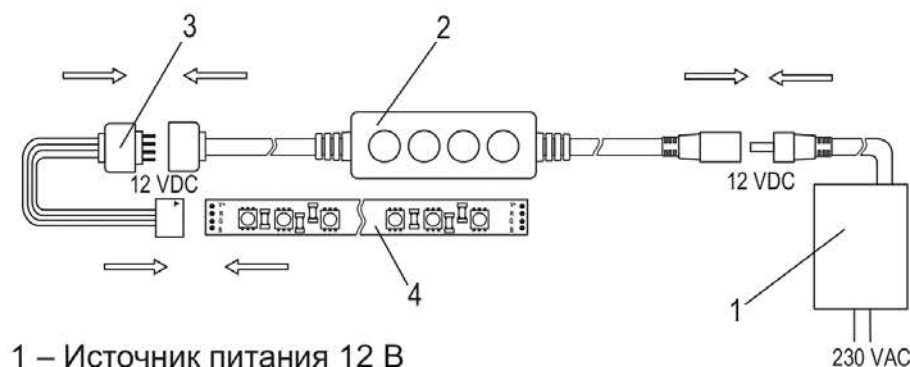
Рисунок 8 – Схема параллельного подключения многоцветной RGB светодиодной ленты к блоку питания и контроллеру
