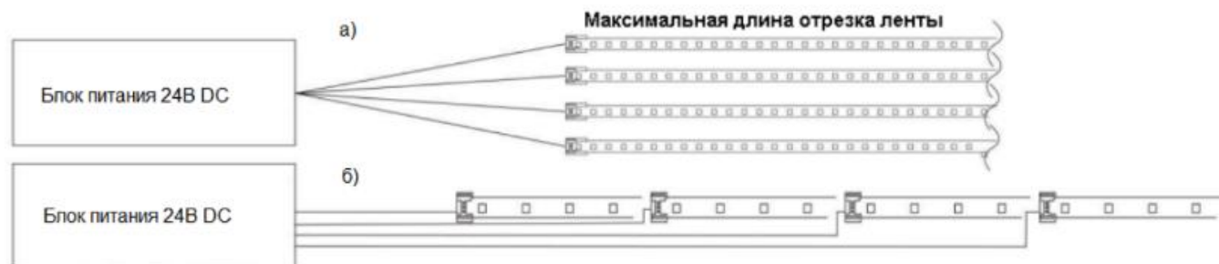
а) Шлейфовое подключение светодиодной ленты; б) подключение нескольких отрезков светодиодной ленты смонтированных в одну линию.
