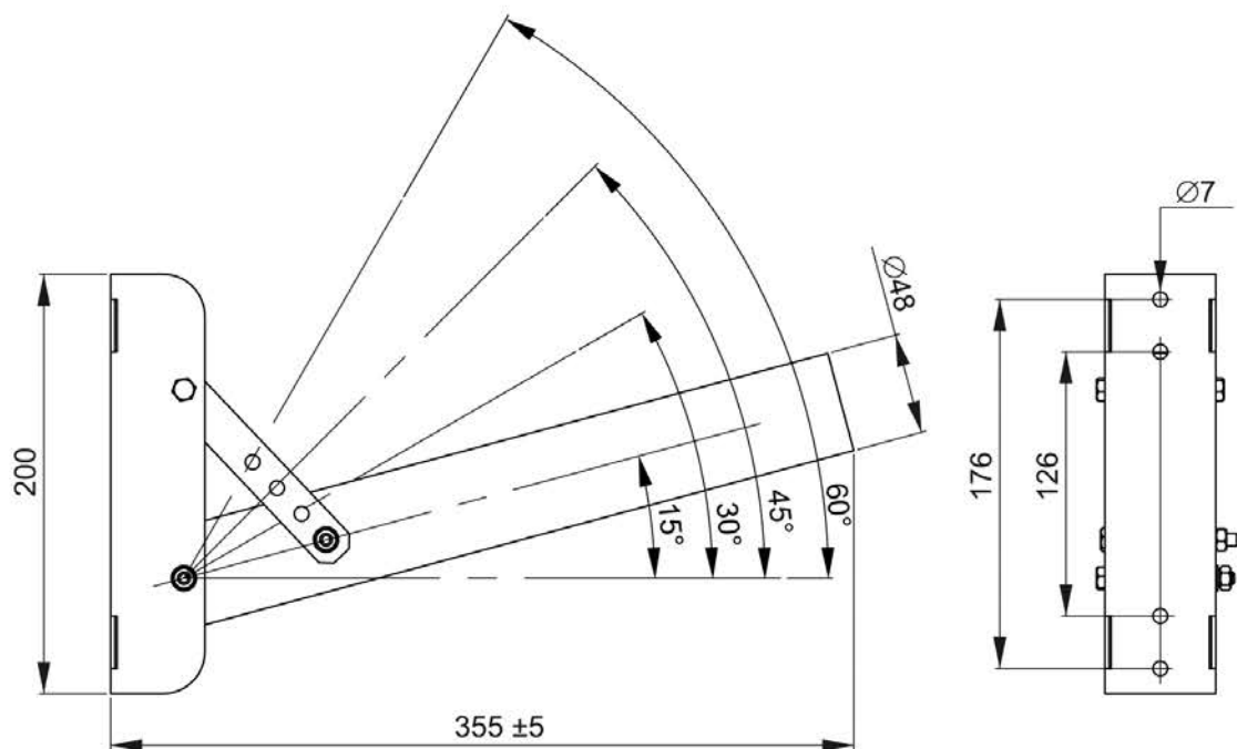
Рисунок 5 – Кронштейн LDKU0D-CR-48-0350-23-K01
