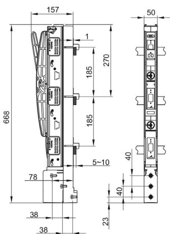
a) ПВР-3 160 А / PVR-3 160 А
