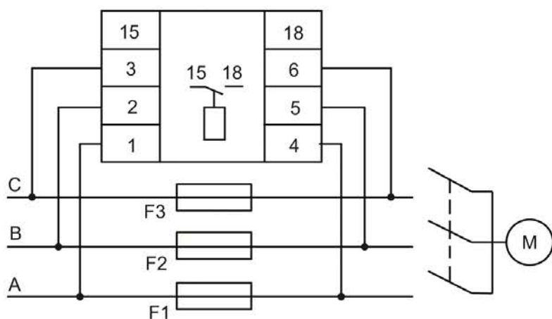
c) РКСП / RKSP
