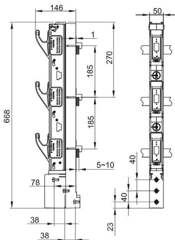
b) ПВР-1 160А / PVR-1 160А
