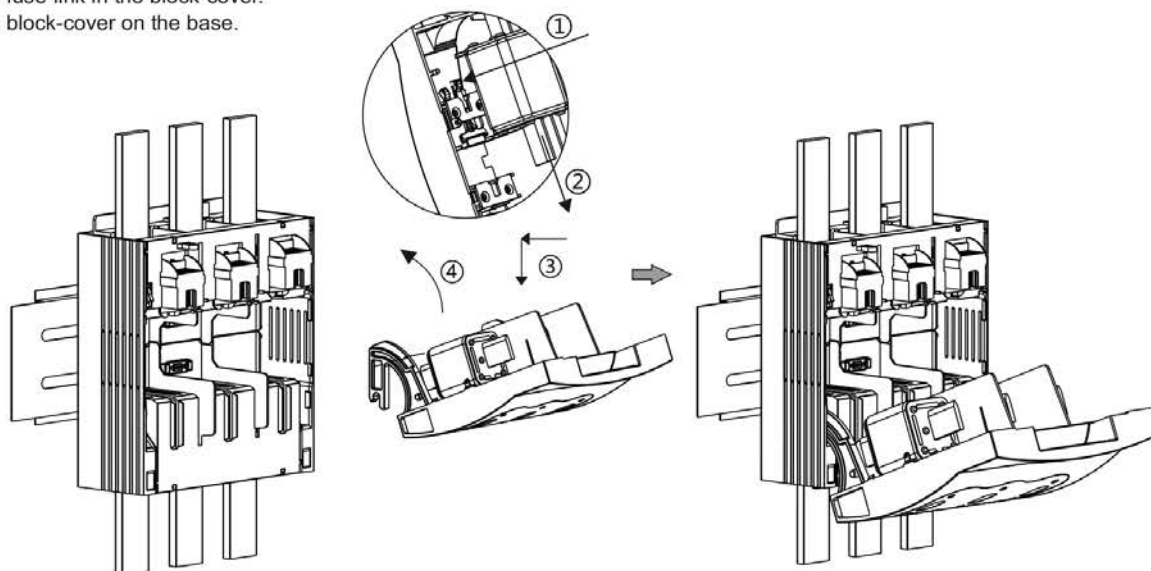
Рисунок 6 – Монтаж горизонтальных ПВР на токи 250–630 A / Figure 6 – Installation of horizontal PVR for 250–630 A currents
