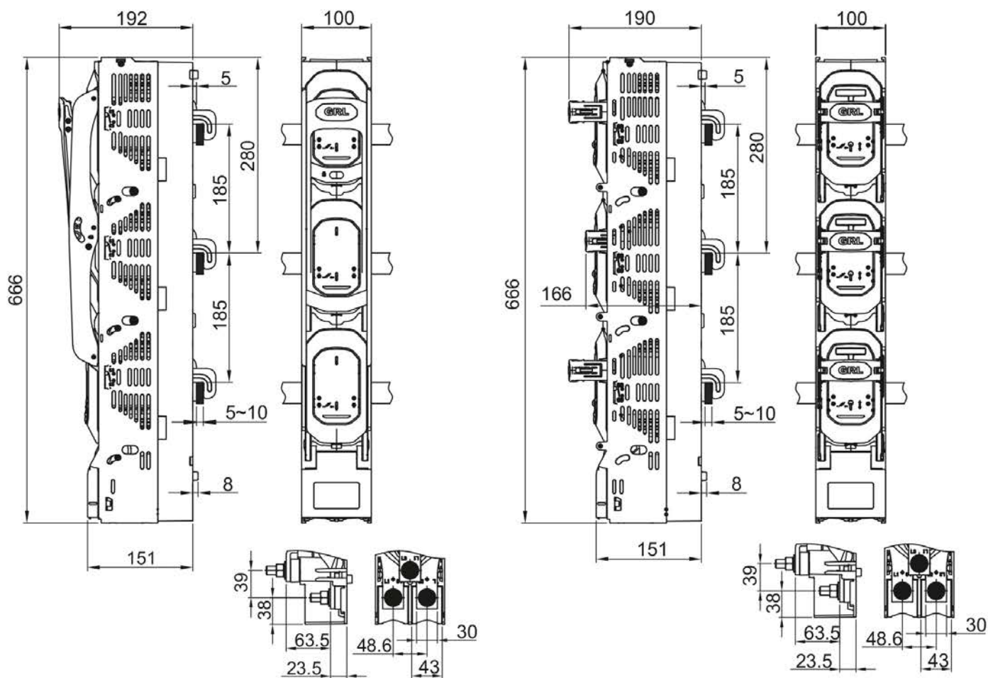
c) ПВР-3 250 - 630 A / PVR-3 250 – 630 A
