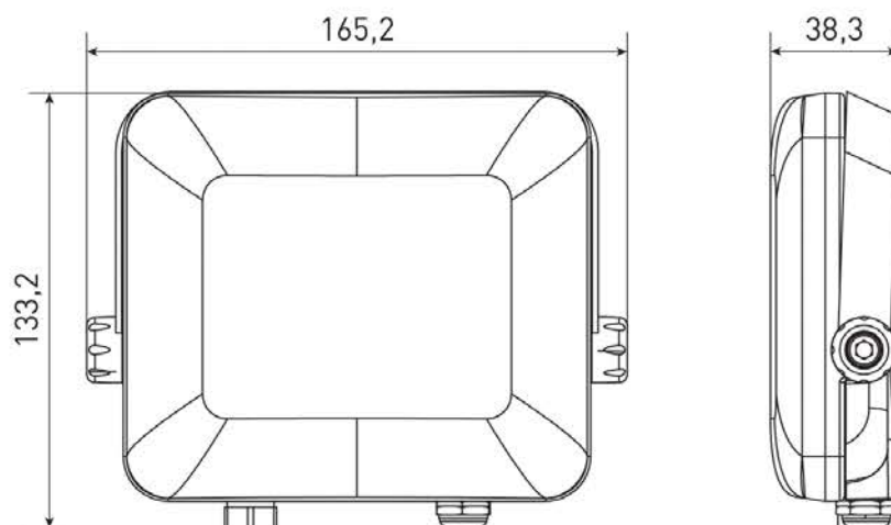
Рис. 3. Габаритные размеры прожекторов мощностью 30 Вт
