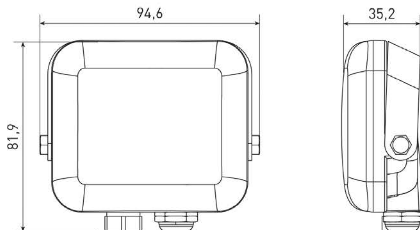
Рис. 1. Габаритные размеры прожекторов мощностью 10 Вт
