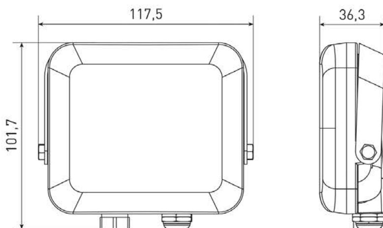
Рис. 2. Габаритные размеры прожекторов мощностью 20 Вт
