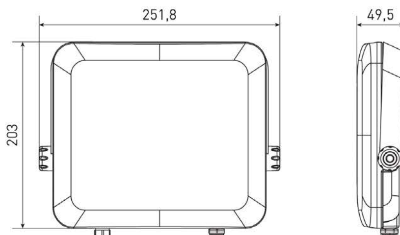
Рис. 5. Габаритные размеры прожекторов мощностью 100 Вт
