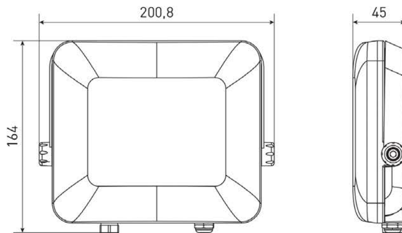
Рис. 4. Габаритные размеры прожекторов мощностью 50 Вт
