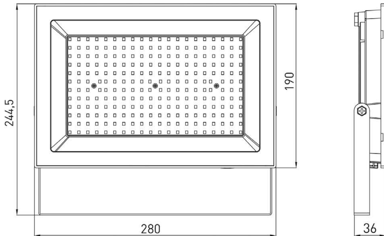
Рис. 7. Габаритные размеры прожекторов мощностью 150 Вт
