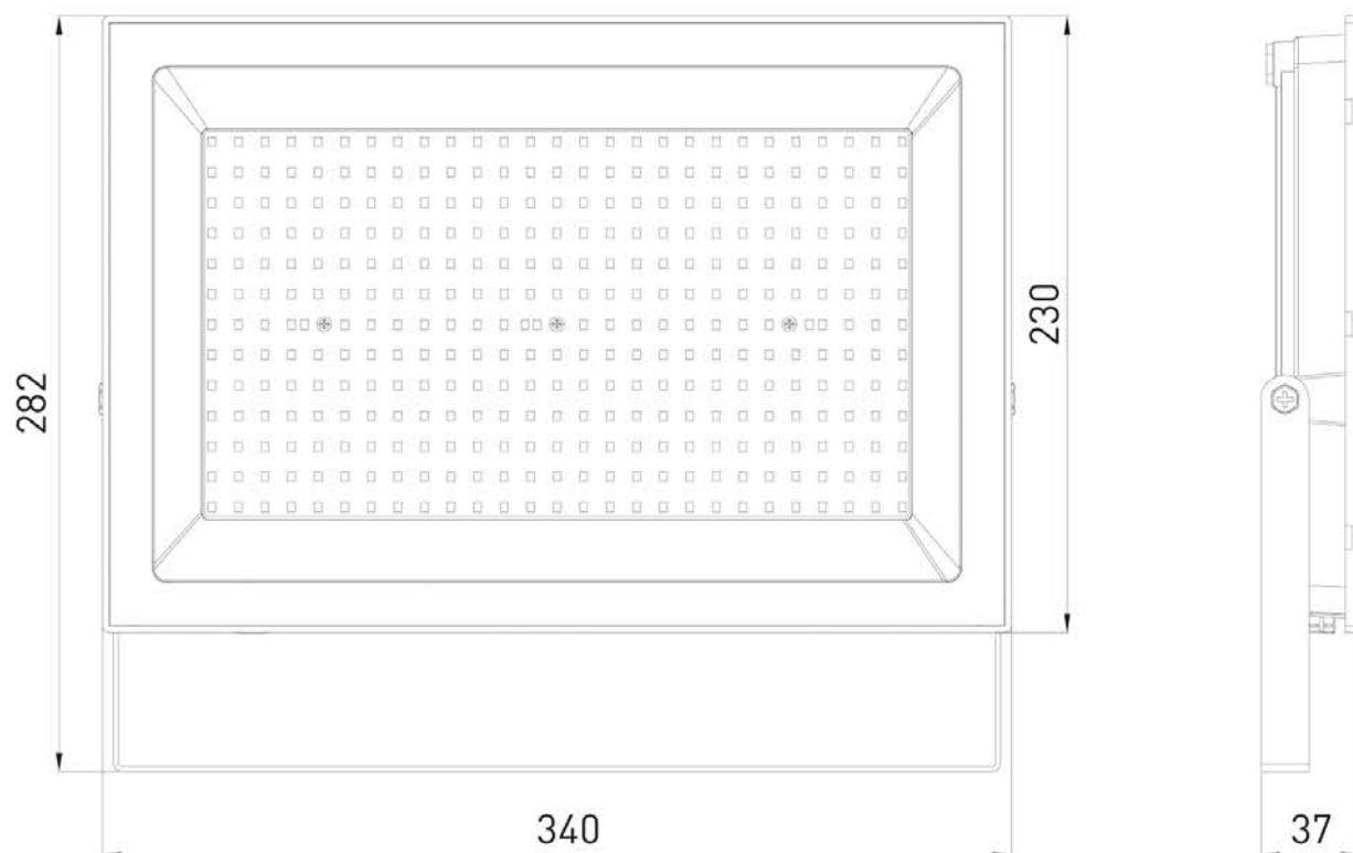
Рис.8. Габаритные размеры прожекторов мощностью 200 Вт
