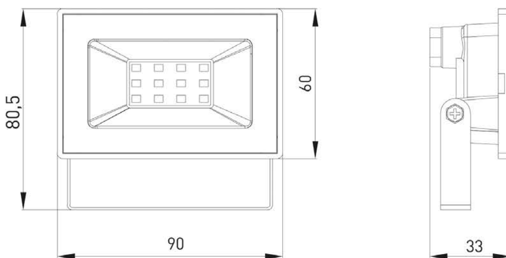
Рис. 2. Габаритные размеры прожекторов мощностью 20 Вт
