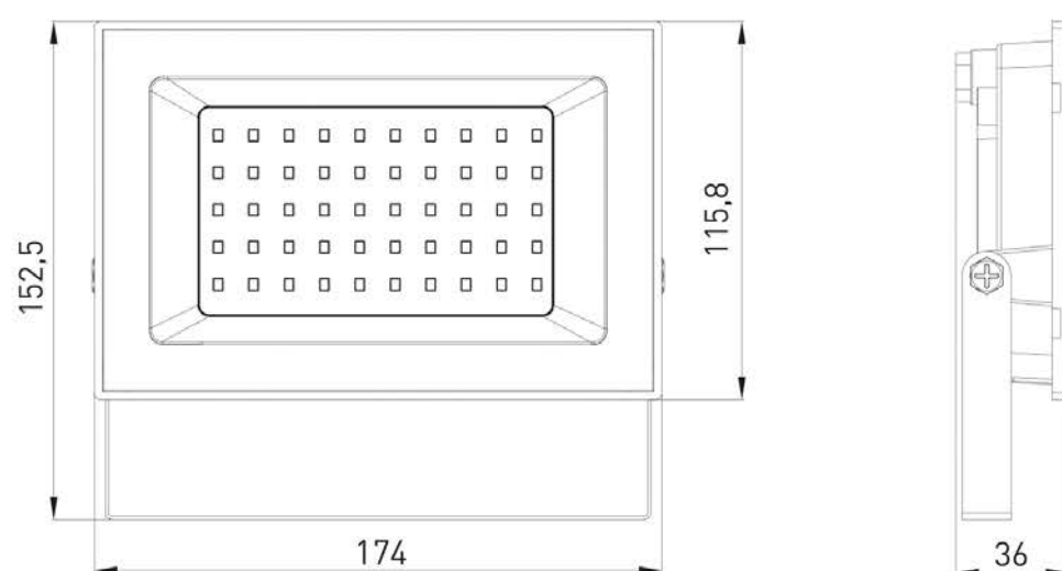
Рис. 5. Габаритные размеры прожекторов мощностью 75 Вт
