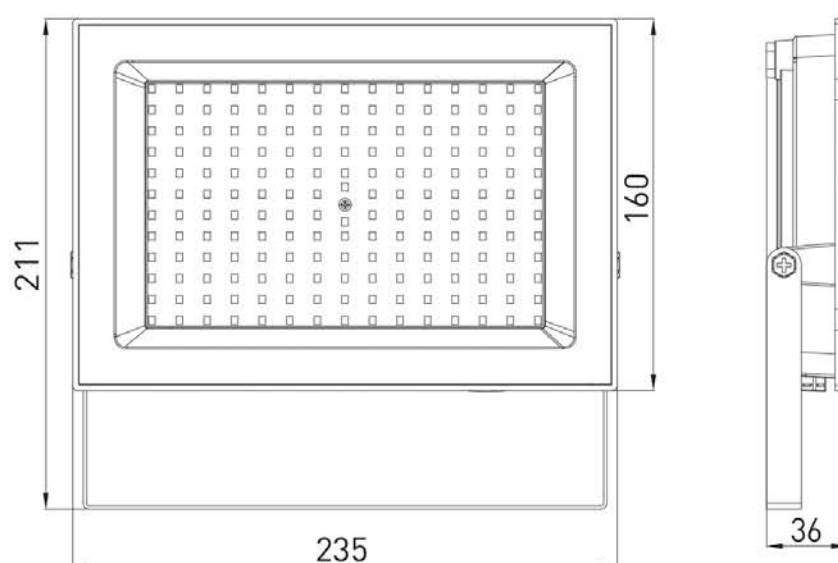
Рис. 6. Габаритные размеры прожекторов мощностью 100 Вт
