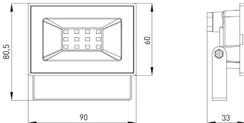
Рис. 1. Габаритные размеры прожекторов мощностью 10 Вт
