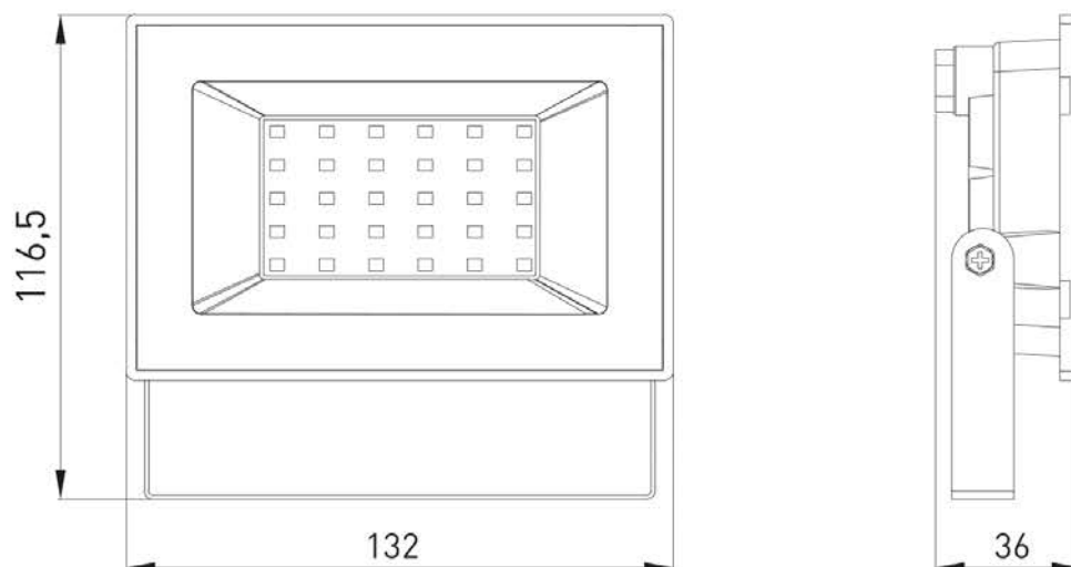
Рис. 4. Габаритные размеры прожекторов мощностью 50 Вт
