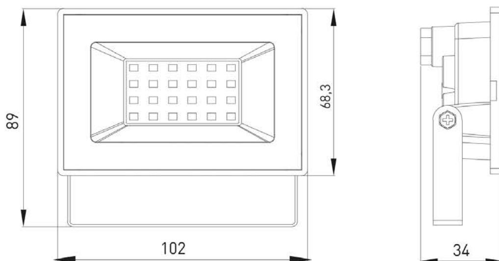
Рис. 3. Габаритные размеры прожекторов мощностью 30 Вт
