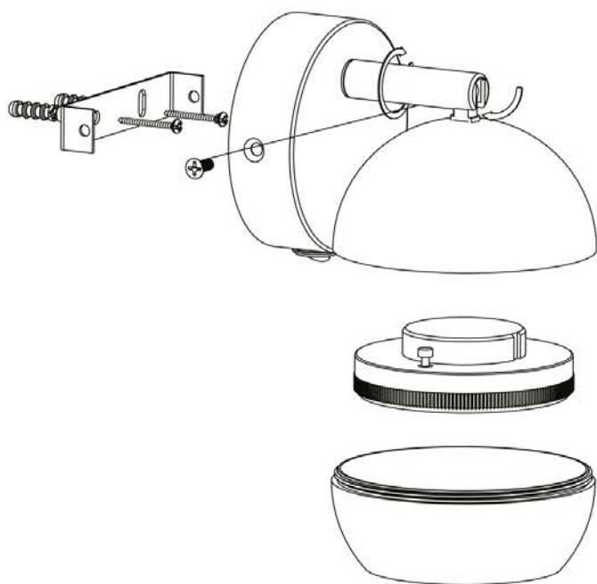
Рисунок 2 – Схема монтажа светильника 4013
