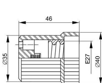
Рисунок 8 – Пкр27-04-K43
