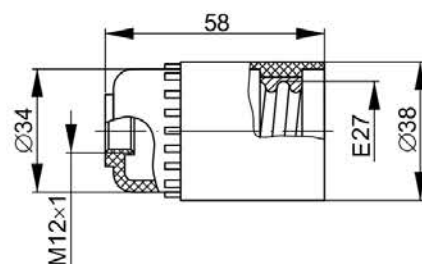
Рисунок 3 – Пк627-04-K01
