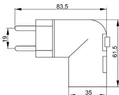
Рисунок 27 – Переходник ПР7/16-27-R02
