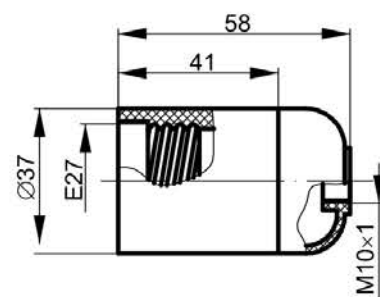
Рисунок 12 – Ппл27-04-K02
