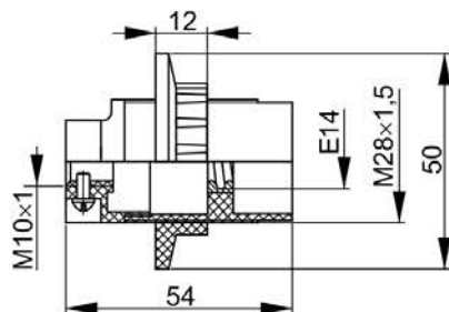
Рисунок 5 – Пк614-04-K11
