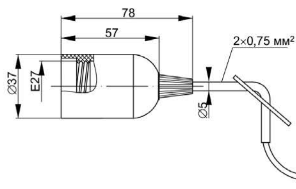
Рисунок 14 – Ппл27-04-K51; Ппл27-04-K52
