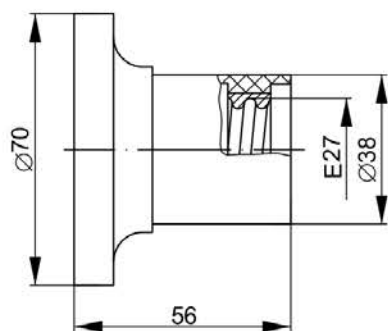
Рисунок 4 – Пк627-04-K21
