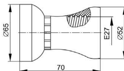
Рисунок 24 – Ппл27-04-K21
