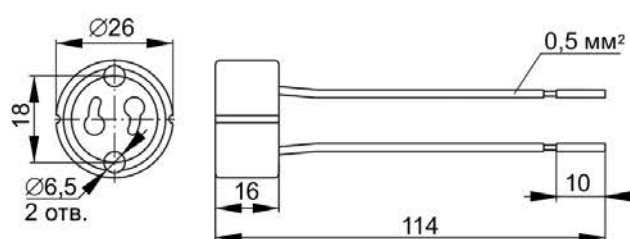
Рисунок 22 – Пкр10-04-K52
