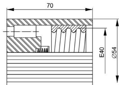
Рисунок 9 – Пкр40-16-K43
