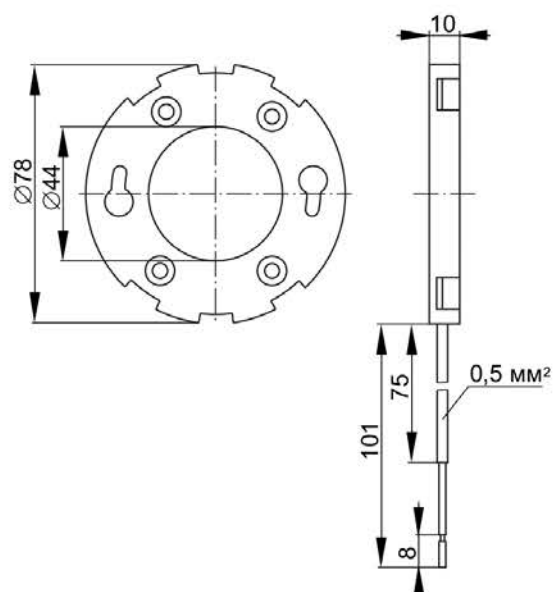
Рисунок 19 – Ппл53-04-K52
