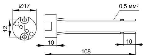
Рисунок 21 – Пкр15-04-K52
