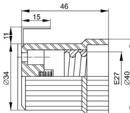
Рисунок 26 – Ппл27-04-K31
