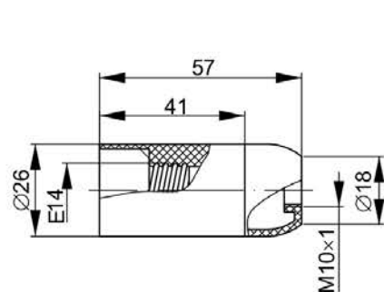
Рисунок 10 – Ппл14-02-K02
