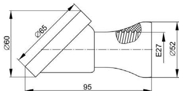
Рисунок 23 – Ппл27-04-K31
