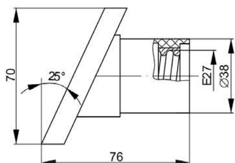
Рисунок 1 – Пк627-04-K31
