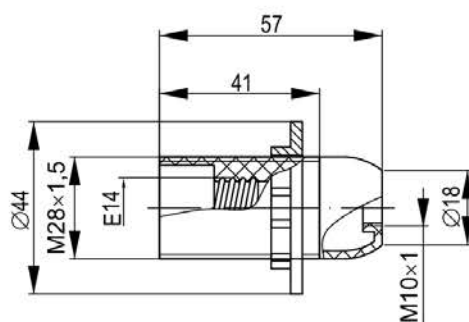
Рисунок 11 – Ппл14-02-K12
