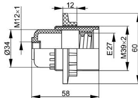
Рисунок 6 – Пк627-04-K11
