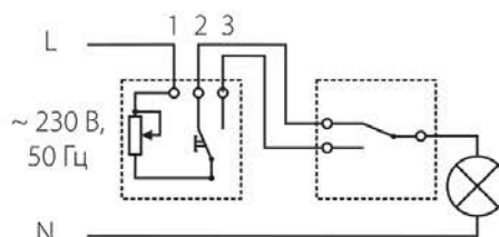
Подключение диммера с проходным выключателем
