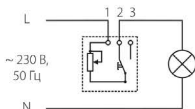
Схема подключения диммера
