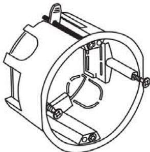
Подрозетник
