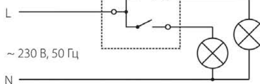
Двухклавишный выключатель
