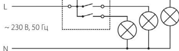
Трехклавишный выключатель
