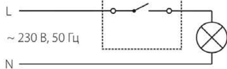
Одноклавишный выключатель
