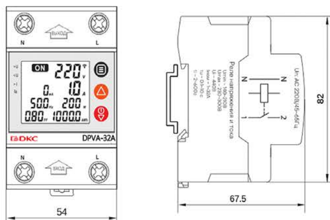
Рисунок 4 – Габаритные размеры реле DPVA
