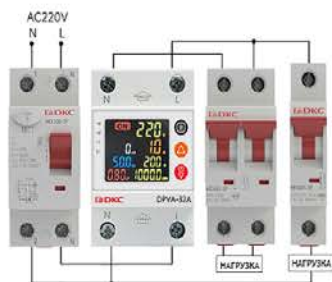
Рисунок 6 – Схема подключения реле DPVA
