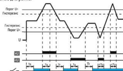
Рисунок 7 – Функциональная диаграмма перенапряжения и понижения напряжения реле DPVA При возникновении ошибки перенапряжения/пониженного напряжения устройство защиты выключится. Когда напряжение вернется в норму, устройство защиты включится через время сброса, а значение перенапряжения/пониженного напряжения может быть заново установлено.
