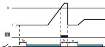
Рисунок 8 – Функциональная диаграмма перегрузки по току реле DPVA Когда текущее значение превысит установленное значение тока и продлится в течение времени T<sub>с</sub>, защита выключится и начнет сброс с задержкой T<sub>р</sub>. По истечении времени сброса она снова включится.
