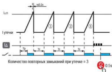
Рисунок 9 – Функциональная диаграмма тока утечки реле DPVA Когда ток утечки в цепи превысит установленное значение, устройство защиты отключится. Вы можете отключить функцию защиты от утечки. Данный фильтр будет сброшен в соответствии с заданным
