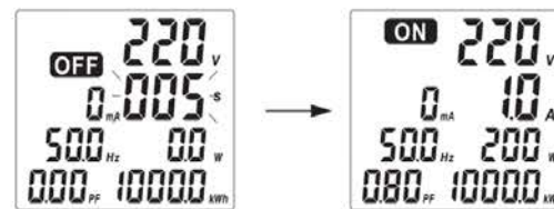
Рисунок 2 – Внешний вид панели при ручном выключении реле DPVA
