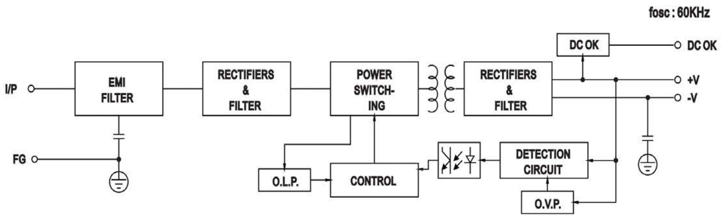
Рис 2. Блок схема DR-M-20W-5/12/24
