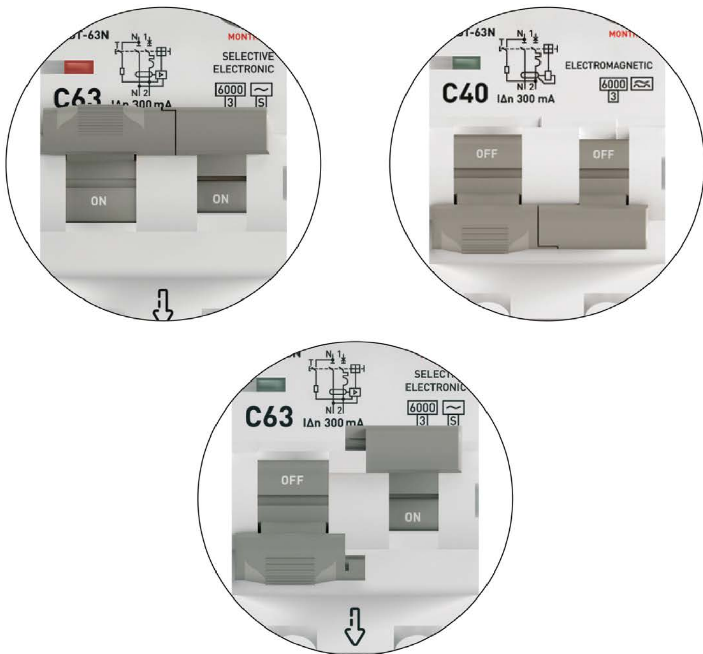
Рис. 7 – Цветовой индикатор состояния контактной группы
