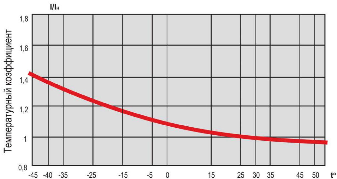
Рис. 2 – Коэффициент пересчета номинального тока в зависимости от температуры окружающей среды
