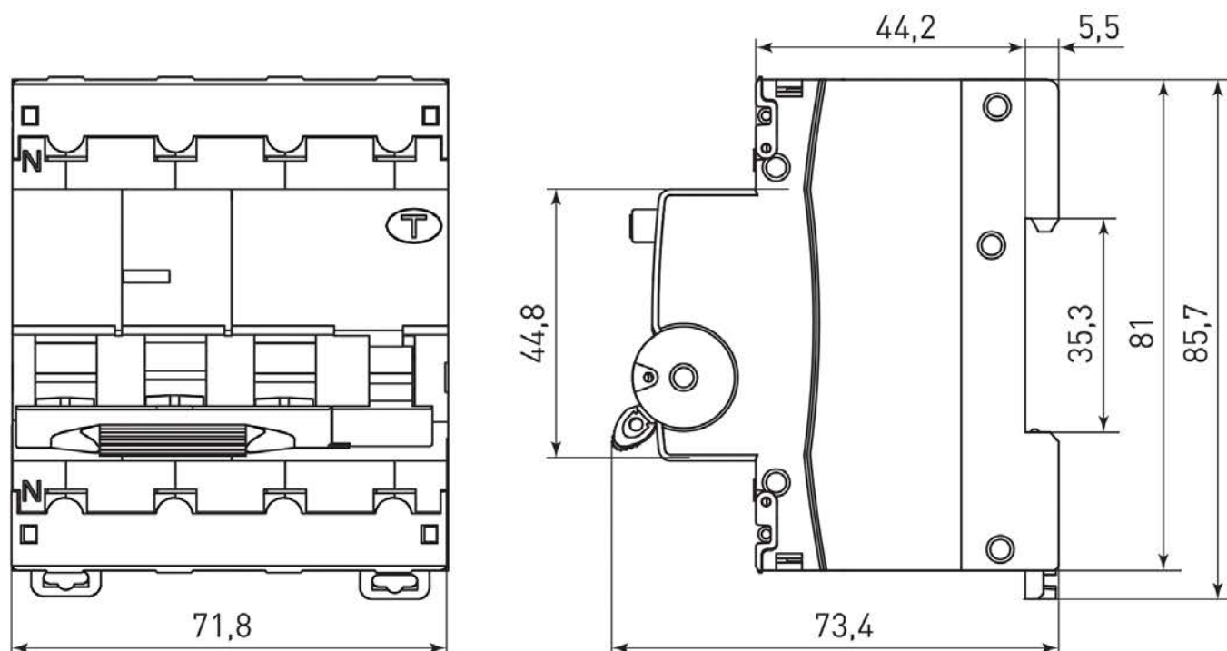
Рис. 36 – Габаритные размеры АВДТ-63N 3P+N
