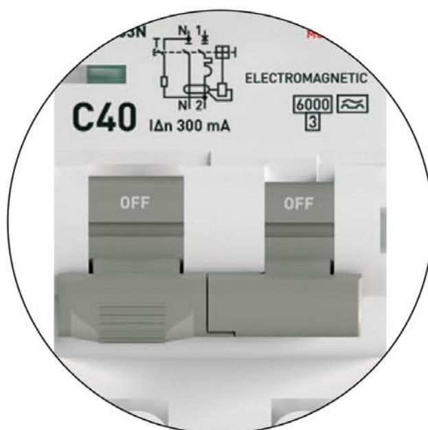
Рис. 6 – Индикация срабатывания АВДТ-63N по току утечки
