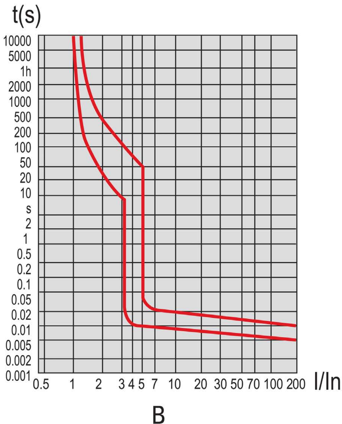
Рис. 1а – Время-токовые характеристики
