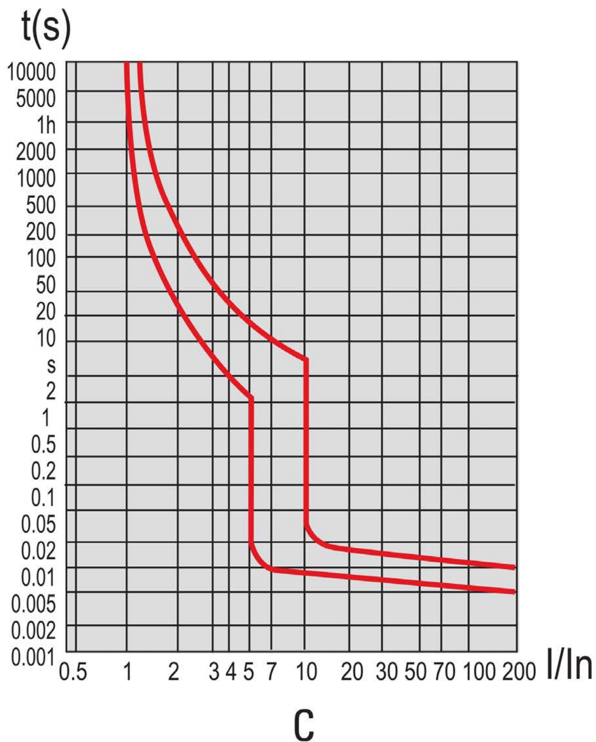
Рис. 16 – Время-токовые характеристики
