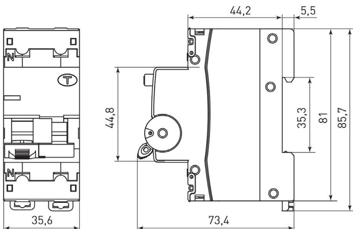
Рис. 3а – Габаритные размеры АВДТ-63N 1P+N
