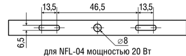
Рис. 2. Размеры лиры, указаны в мм
