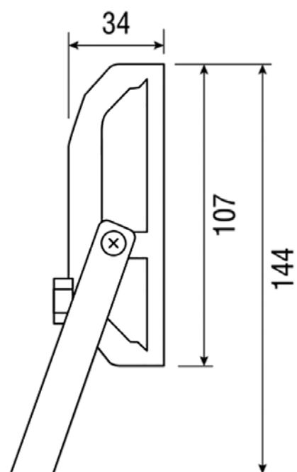
Рис. 3. Установка
