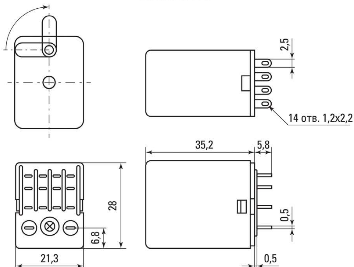
Рис. 5 - Габаритные размеры реле промежуточное RPA 22/4 5A AVERES EKF
