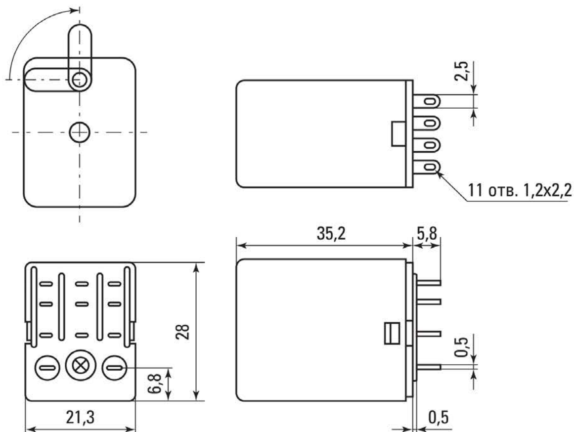
Рис. 4 - Габаритные размеры реле промежуточное RPA 22/3 10A AVERES EKF
