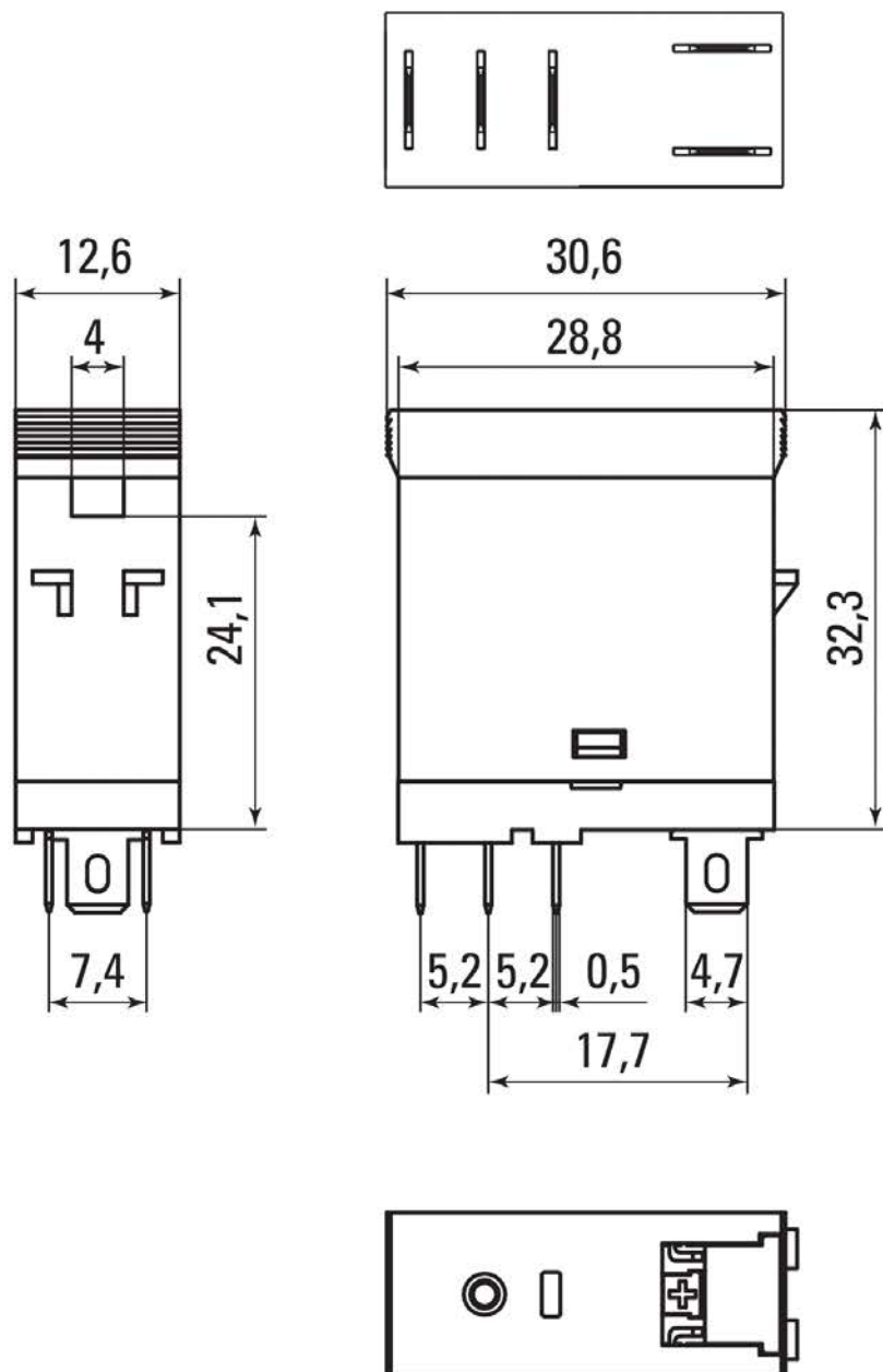
Рис. 2 - Габаритные размеры реле промежуточное RPA(t) 25/1 AVERES EKF
