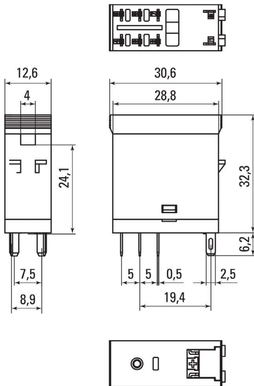
Рис. 3 - Габаритные размеры реле промежуточное RPA(t) 22/2 AVERES EKF
