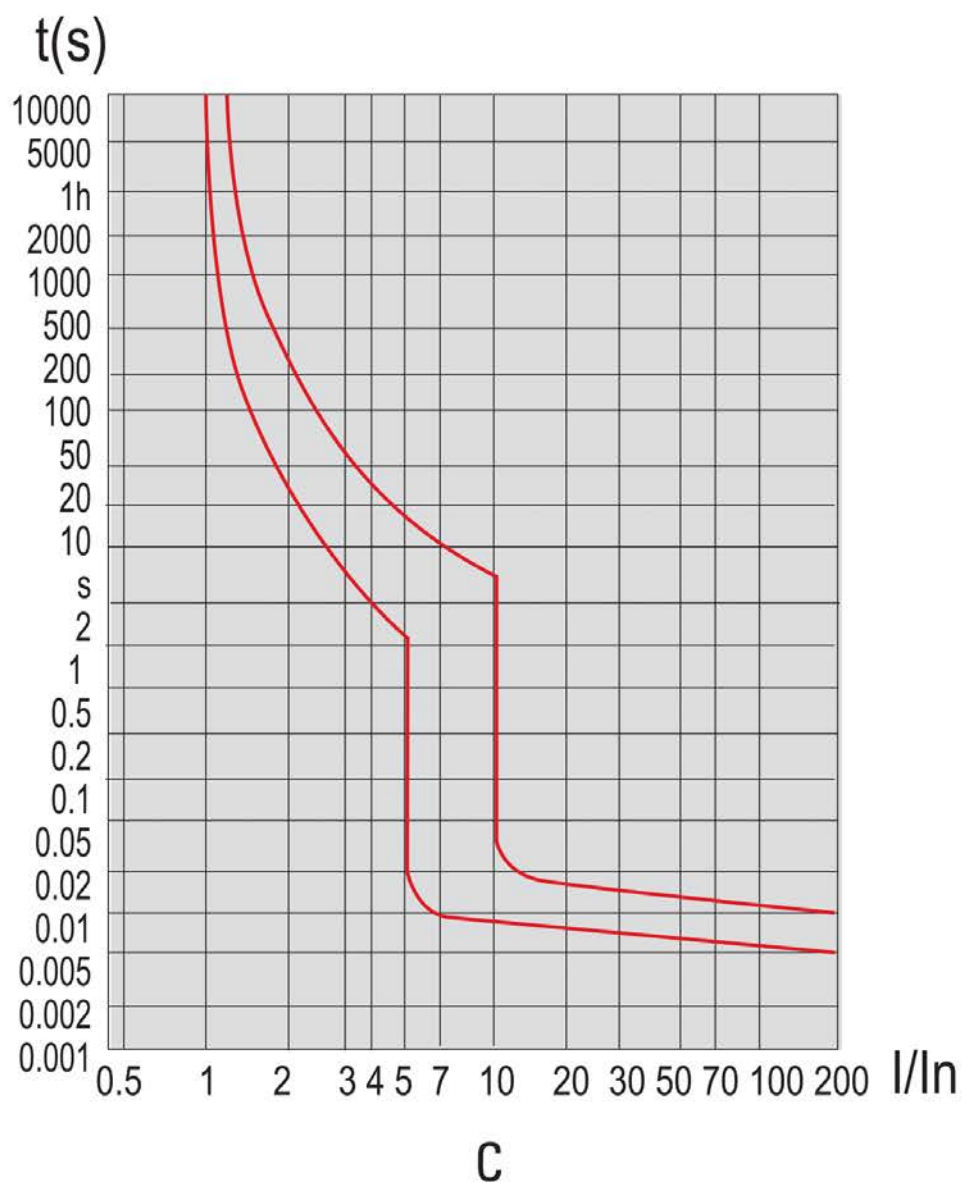
Рис. 2 – Время-токовые характеристики
