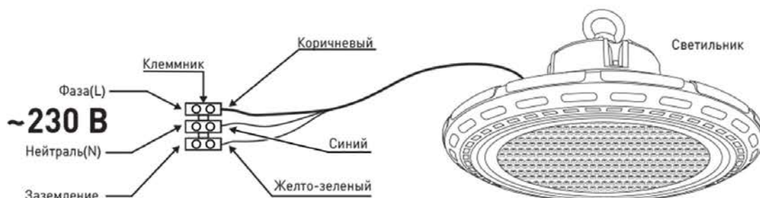
Рис.1. Схема подключения светильника к сети 230В.
