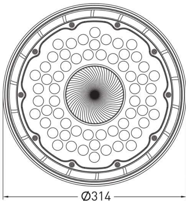
Рис. 3 - Габаритные размеры светильников ДСП-1103
