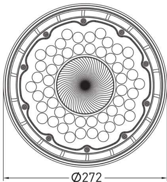
Рис. 2 - Габаритные размеры светильников ДСП-1102
