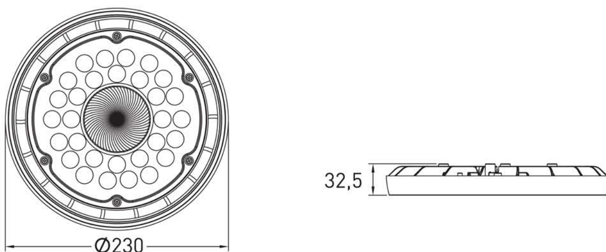
Рис. 1 - Габаритные размеры светильников ДСП-1101
