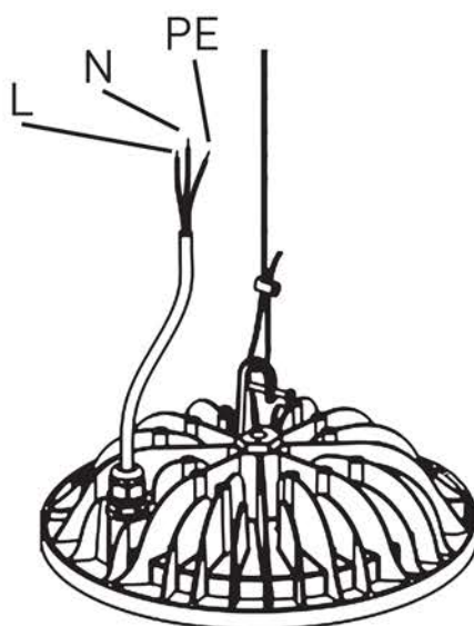
Рис. 4 - Подключение светильника к сети 230 В
