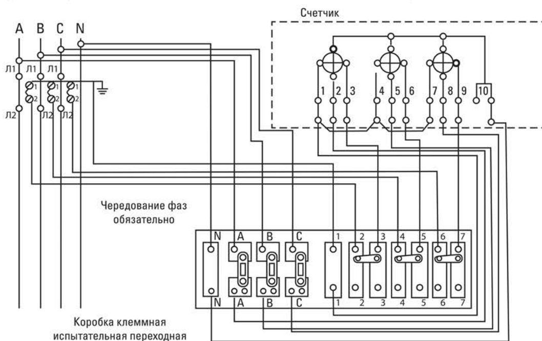
Рис. 1 - Схема подключения трехфазного счетчика с трансформаторным включением к четырехпроводной сети 230/400 (В) через коробку типа ККИ Коробка клеммная испытательная переходная типа ККИ соответствует ГОСТ 31195.2.5-2012 (IEC 60998-2-5:1996).
