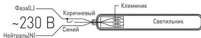
Рис.2. Схема подключения светильника с БАП.
