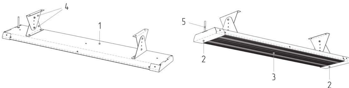
Рисунок 4. Внешний вид и элементы конструкции инфракрасного обогревателя.
