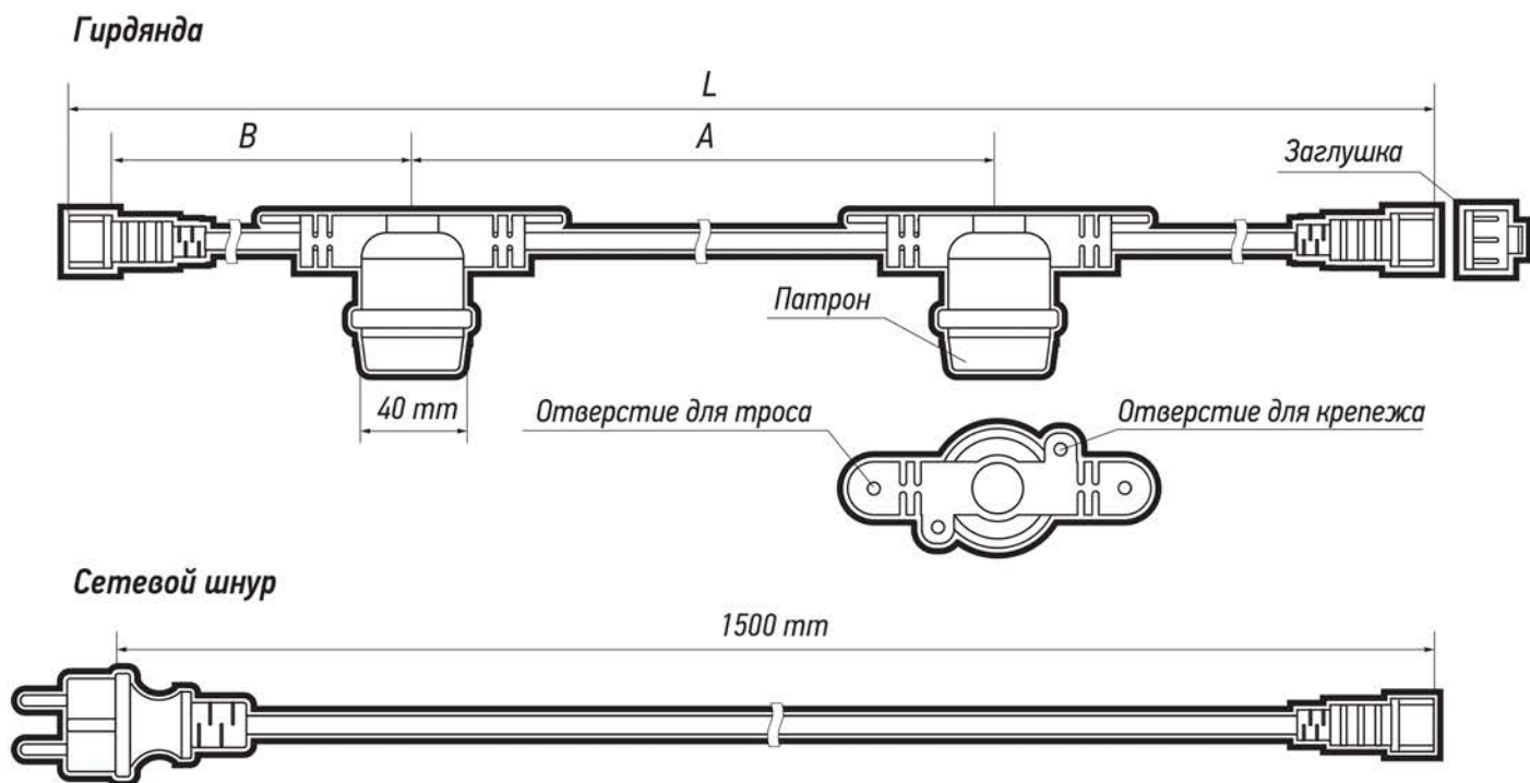
Рис. 1 Гирлянда электрическая белт лайт серии PBL
