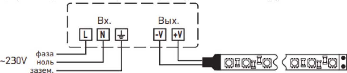
Рисунок 1 – Схема подключения
