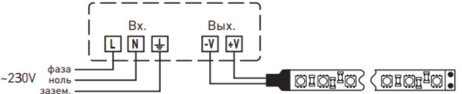
Рисунок 1 – Схема подключения
