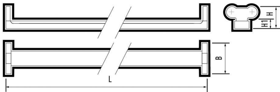
Рис.2 Светильник PPO-T8 2x1200
