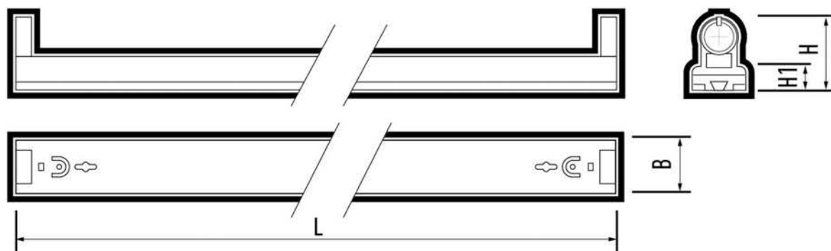
Рис.1 Светильник PPO-T8 1x1200
