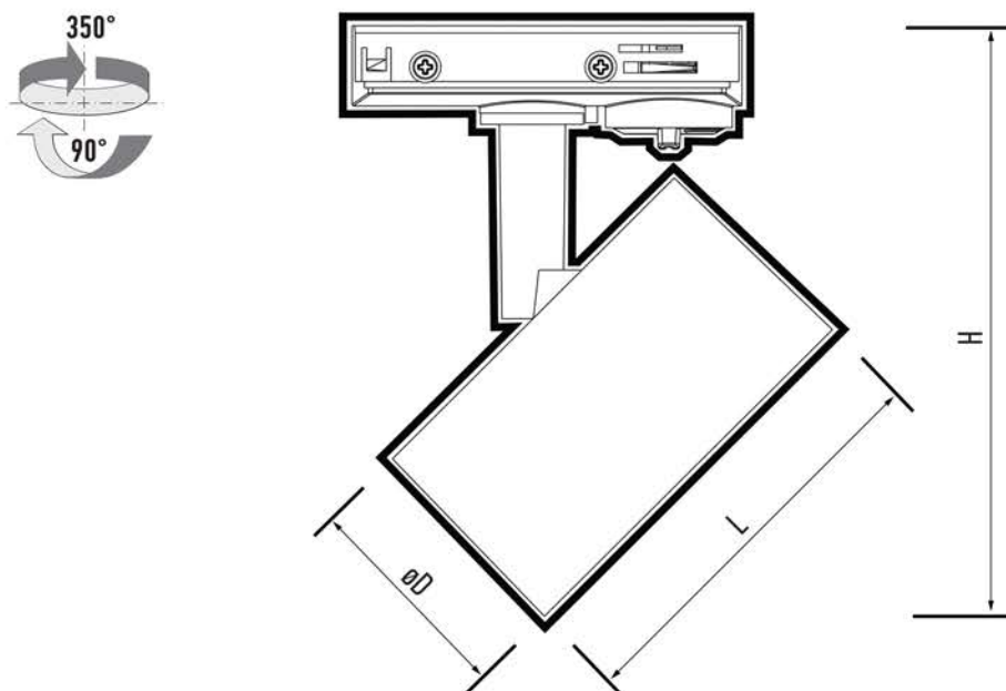
Рис. №1 Светильник PTR 30
