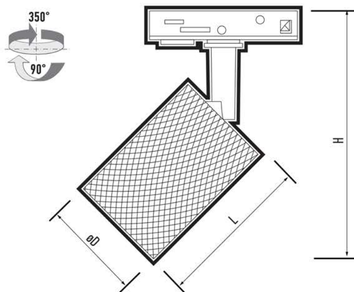
Рис. №1 Светильник PTR 29
