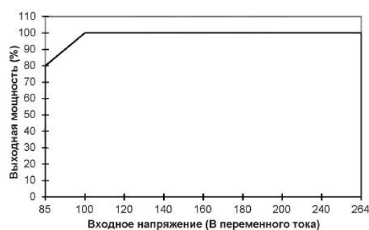
Снижение выходной мощности в зависимости от входного напряжения
