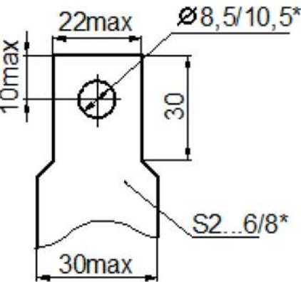
Форма и размеры присоединяемой шины
