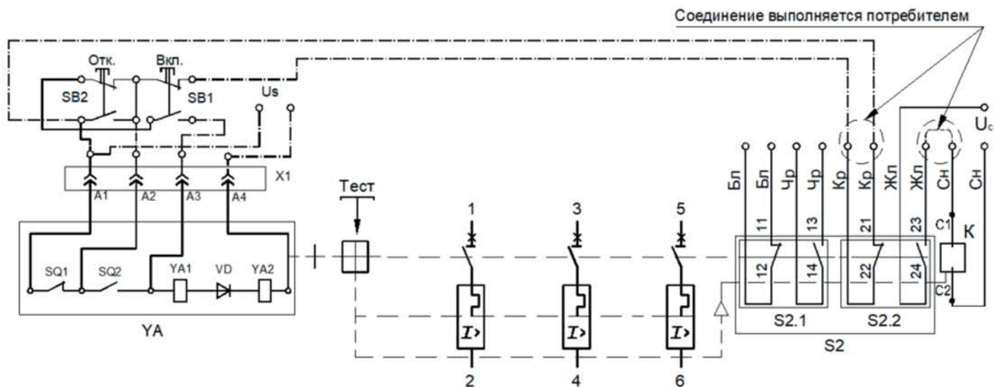
Рисунок В.5 – Схема электрическая принципиальная выключателей с электромагнитным приводом, с независимым расцепителем и вспомогательными контактами
