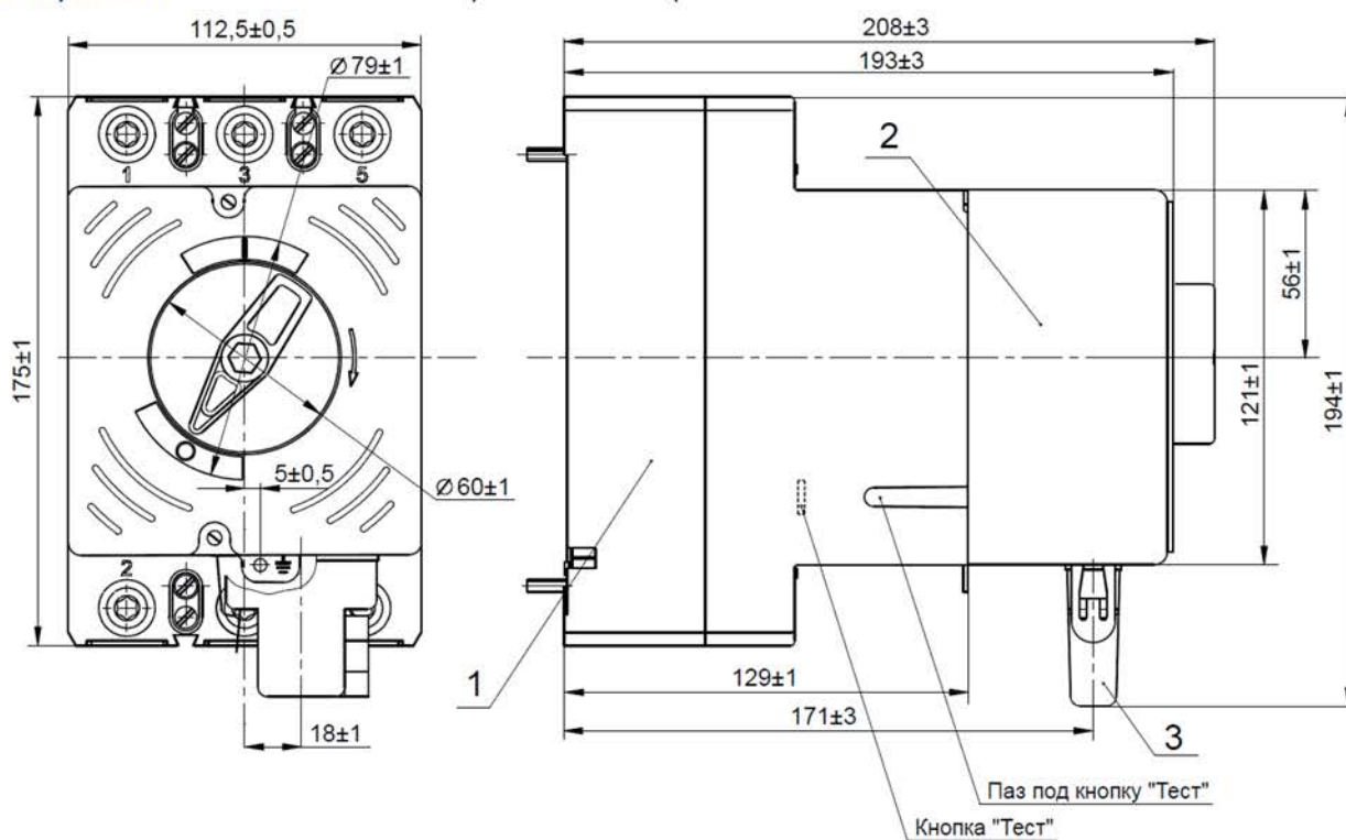
Рисунок Б.3 – Выключатель с электромагнитным приводом
