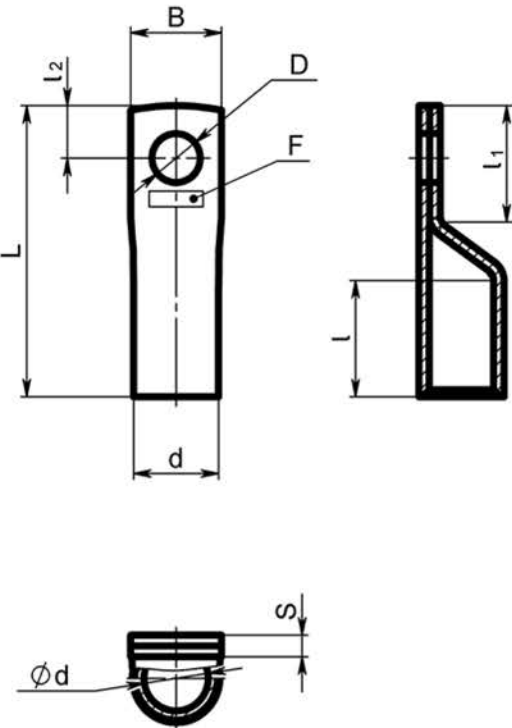
Форма и размеры присоединяемой шины
