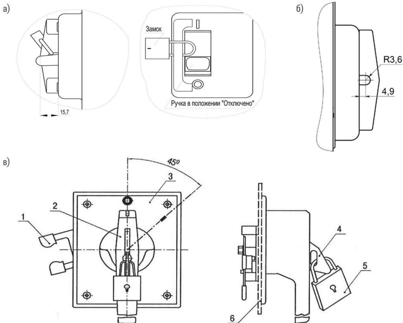
Рисунок 2 – Запирающее устройство в положении «Отключено»
