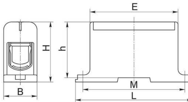
Рисунок 3 - KCB 35-240
