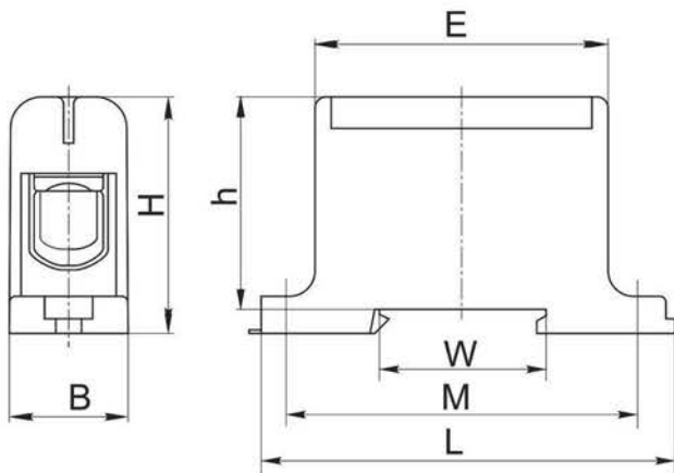
Рисунок 2 - KCB 16-95 (1/2), KCB 35-150
