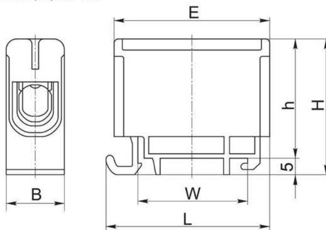
Рисунок 1 - КСВ 6-50 (/2, /3)
