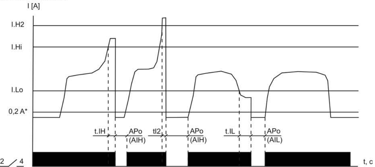
Диаграмма работы реле тока
