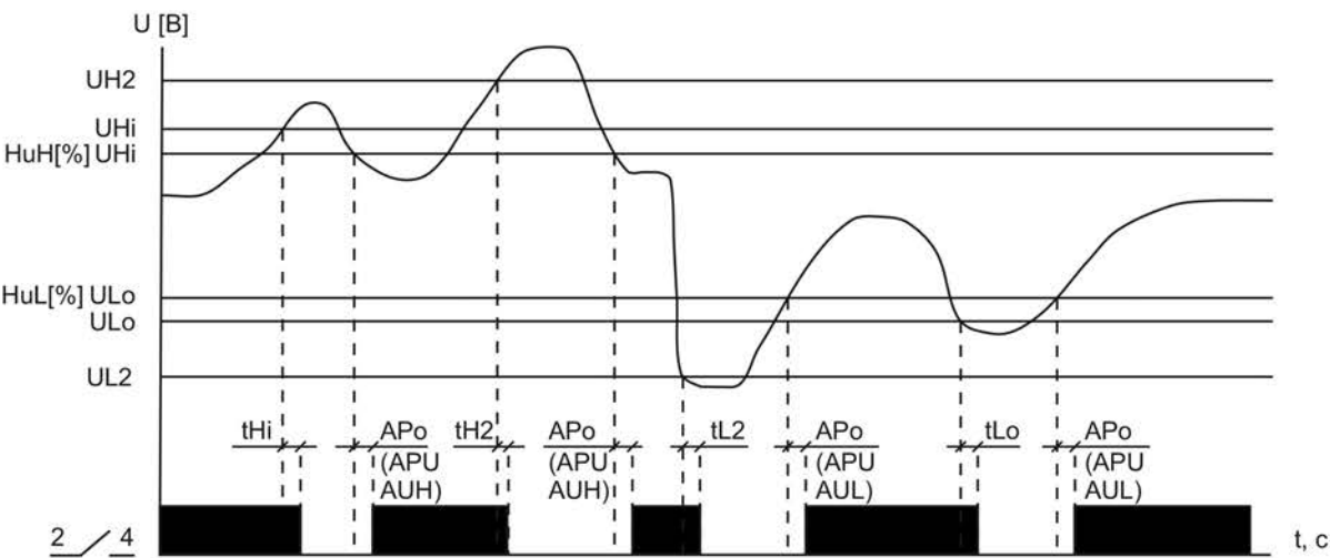
Диаграмма работы реле напряжения
