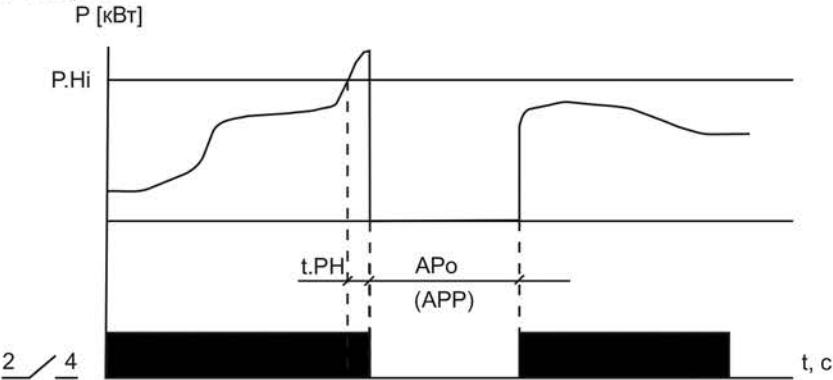
Диаграмма работы реле мощности
