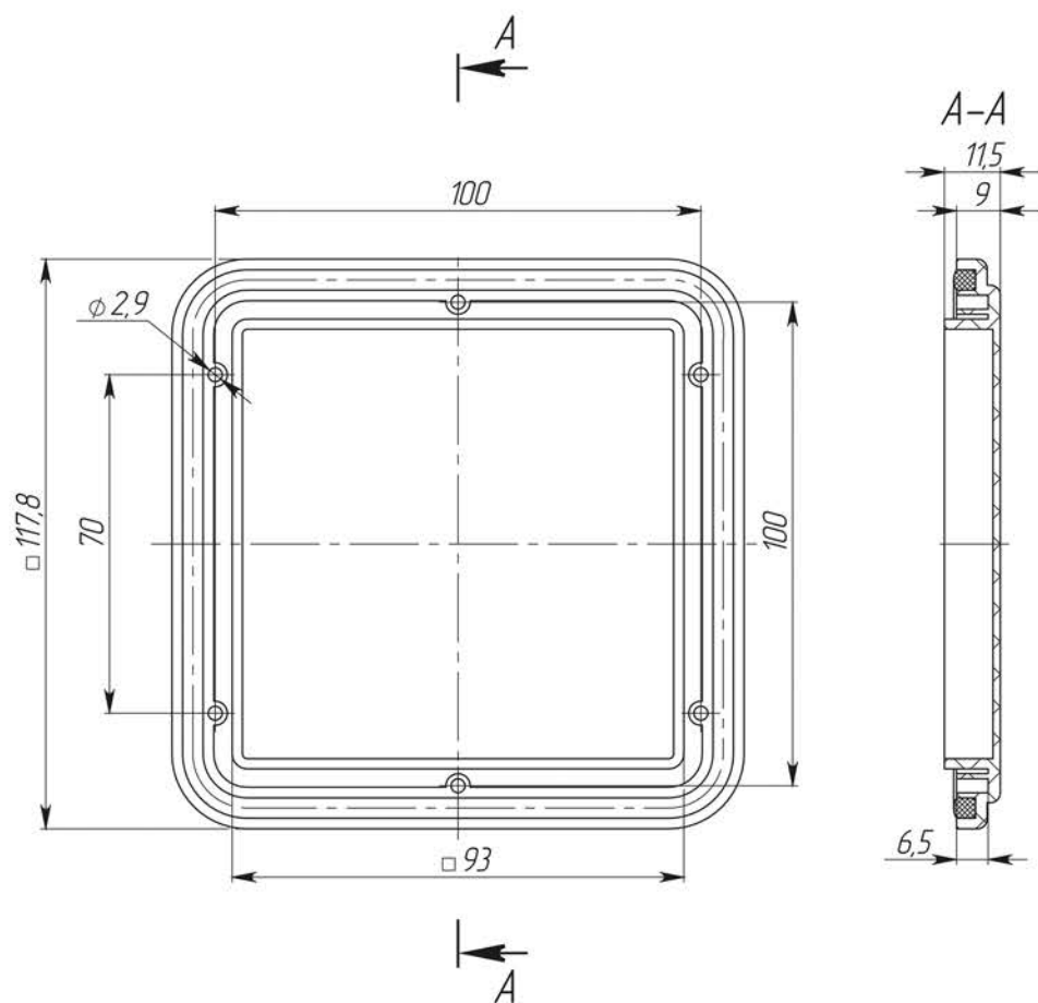
Рисунок / Figure / Сурет 1– Окошко смотровое для корпусов полиэстерных / Sight window for polyester enclosures / Полиэстерлі корпустарға арналған бақылау тексеру терезесі
