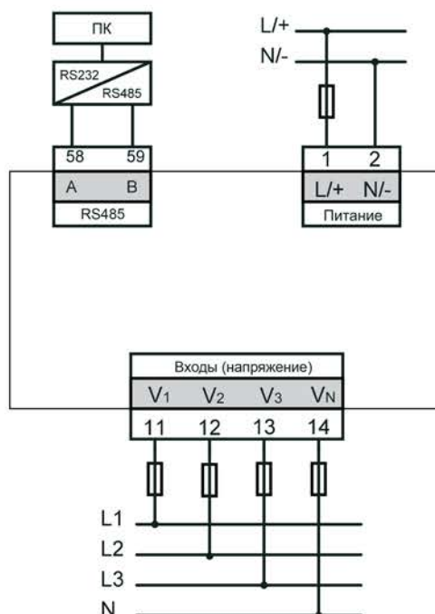
Рисунок 3 — Типовая схема присоединения трехфазного вольтметра
