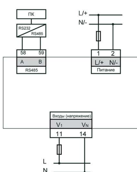
Рисунок 2 — Типовая схема присоединения однофазного вольтметра
