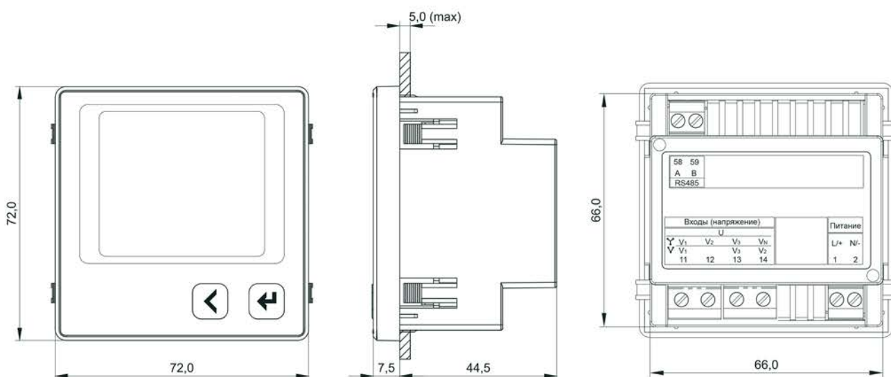
Рисунок 1 — Габаритные размеры вольтметра
