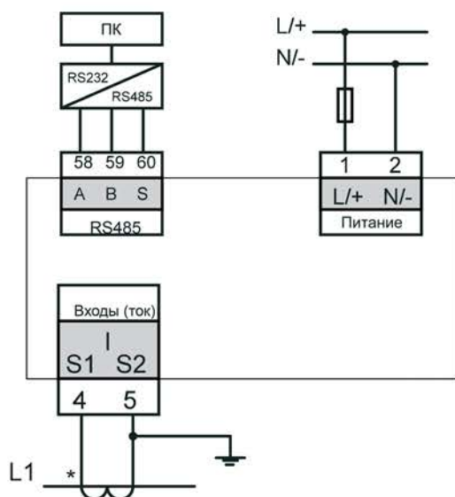
Рисунок 2 — Типовая схема присоединения однофазного амперметра
