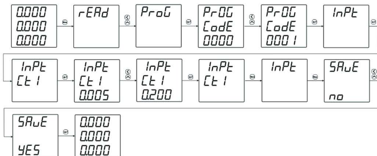
Рисунок 5 — Пример настройки входного сигнала для трехфазного амперметра
