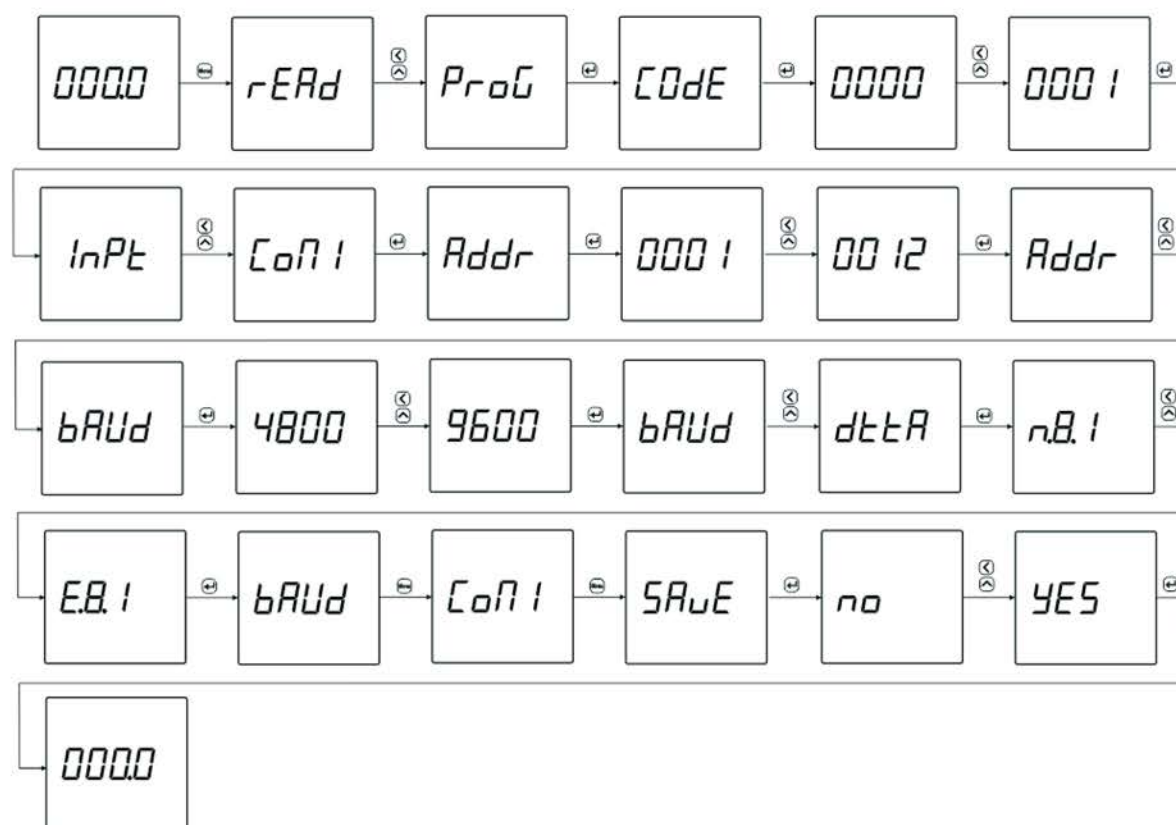
Рисунок 6 — Шаги работы с меню настройки связи
