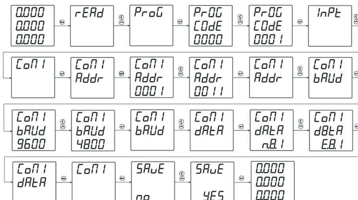
Рисунок 7 — Шаги работы с меню настройки связи
