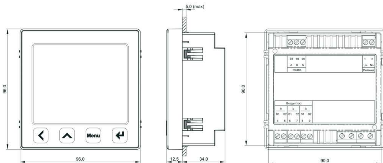
Рисунок 1 — Габаритные размеры амперметра
