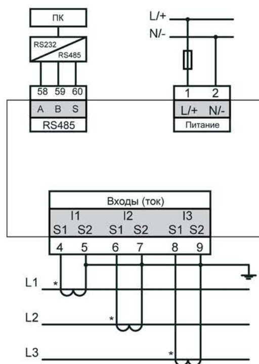
Рисунок 3 — Типовая схема присоединения трехфазного амперметра
