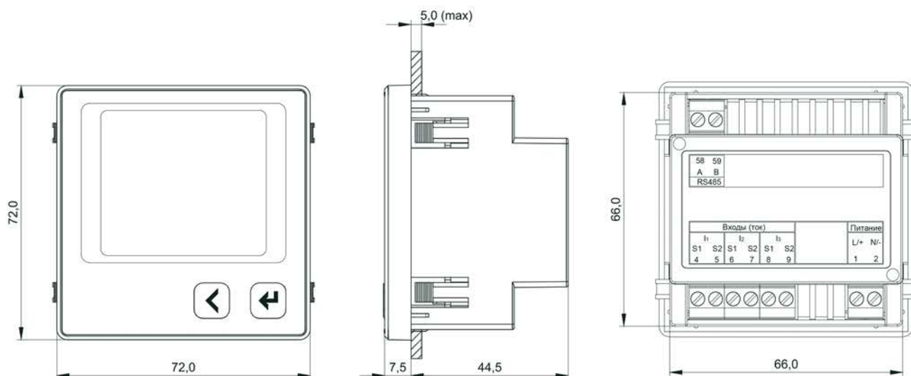
Рисунок 1 — Габаритные размеры амперметра
