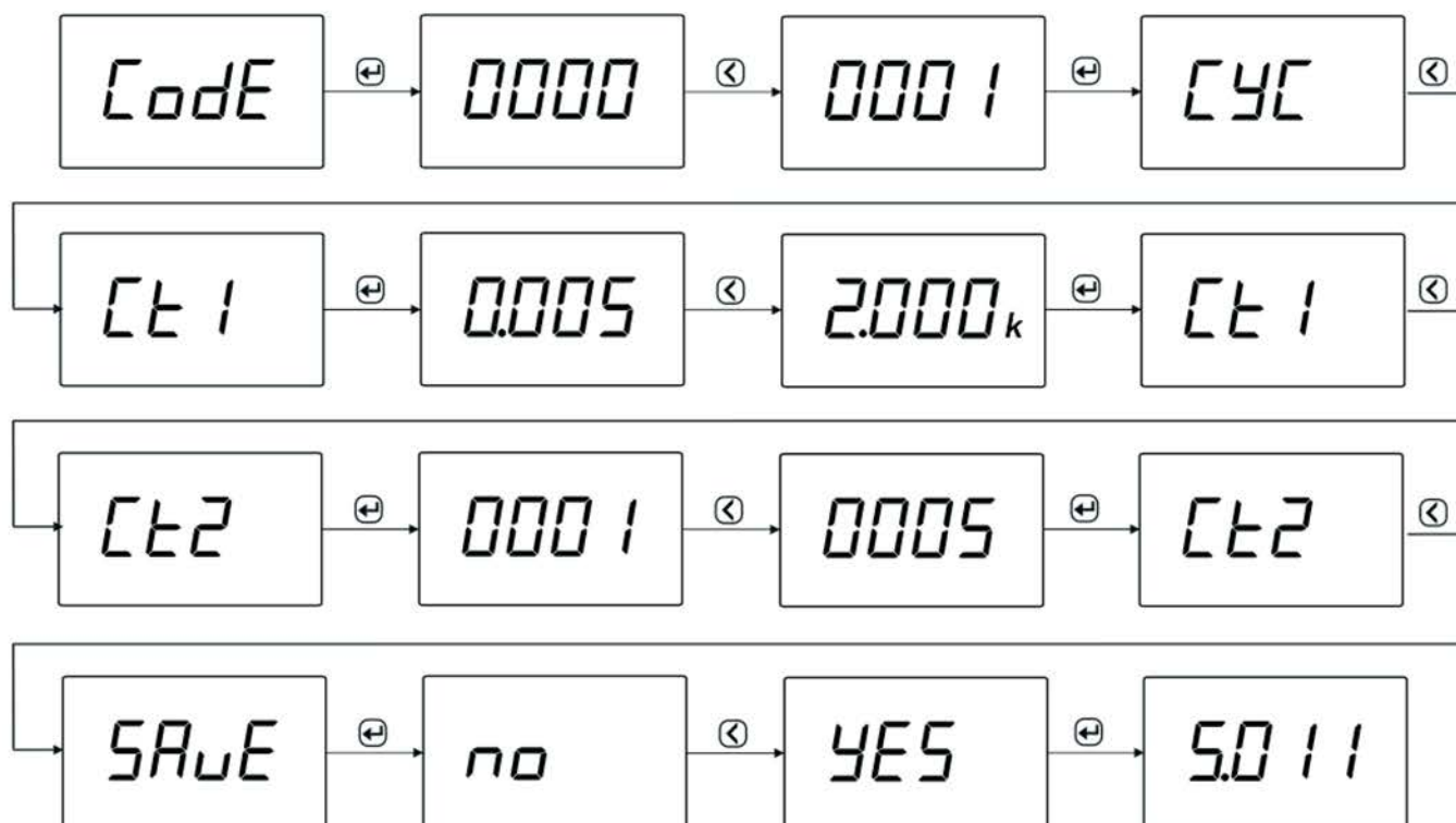
Рисунок 5 — Пример настройки параметра входного сигнала
