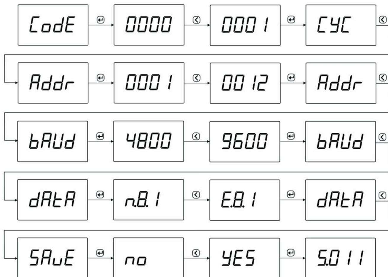
Рисунок 6 — Пример настройки связи
