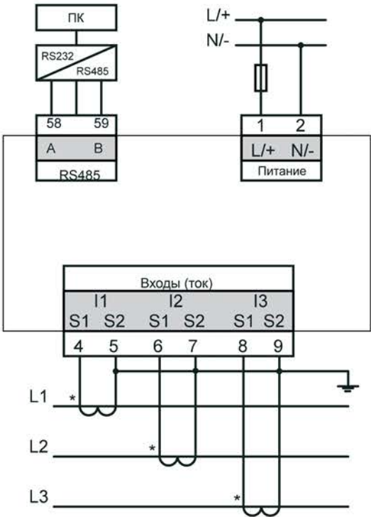
Рисунок 3 — Типовая схема присоединения трехфазного амперметра
