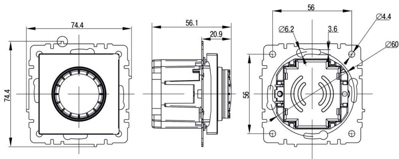
Рисунок 3 – Габаритные размеры диммера / Figure 3 – Overall dimensions of dimmer / 3-сүпет – Диммердің габаритті өлшемдері / Рисунок 3 – Габаритні розміри димеру / 3. attēls – reostata gabarīta izmēri / Pav. 3 – Šviesos regulatoriaus išmatavimai / Joonis 3 – Dimmeri üldmõõtmed / Figura 3 – Dimensiunile variatorului / Bild 3 – Hauptabmessungen des Dimmers
