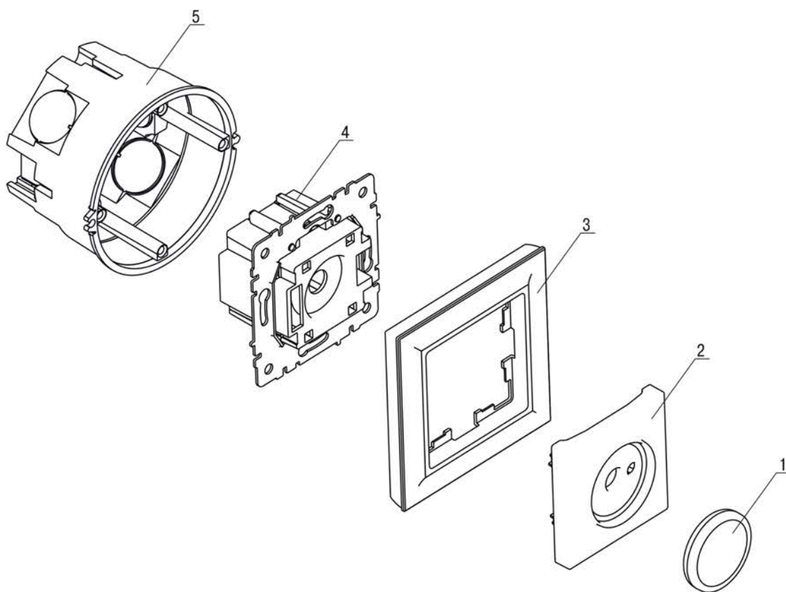
Рисунок 4 – Схема монтажа диммера / Figure 4 – Dimmer mounting diagram / 4-сүпет – Диммерді орнату схемасы / Рисунок 4 – Схема монтажу димера / 4. attēls – reostata uzstādīšanas shēma / Pav. 4 – Šviesos regulatoriaus montavimo schema / Joonis 4 – Dimmeri paigaldamise skeem / Figura 4 – Schema de montare a variatorului / Bild 4 – Montageplan des Dimmers
