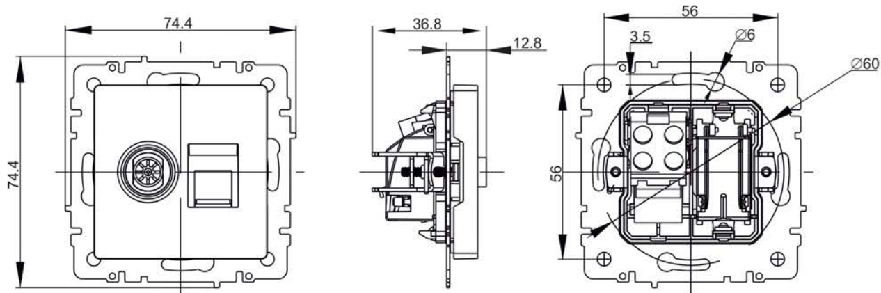
е) PTB/PK12-БрХ*
