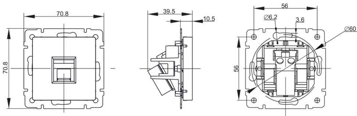
а) PT10-БрХ*
