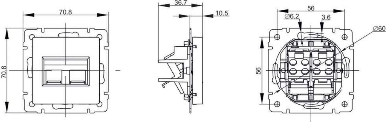
в) PK10-2-БрХ*
