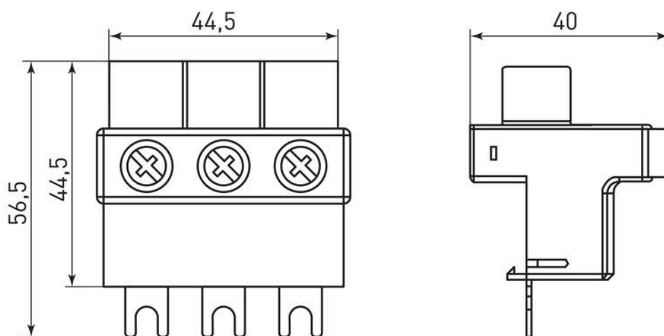
Рис. 6 – Габаритные размеры соединительного блока АПД/GV2 (Артикул: apd-cb)
