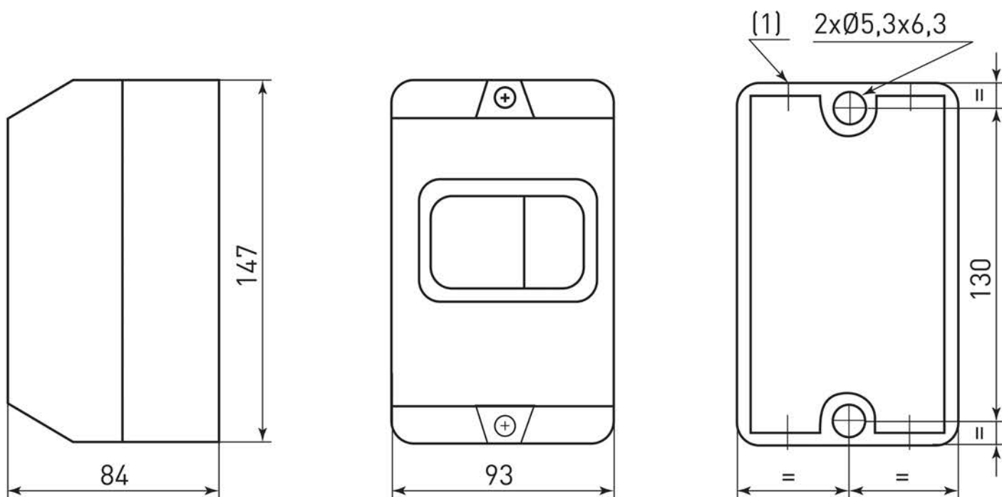
Рис. 2 – Габаритные размеры защитной монтажной коробки (IP41) (Артикул: apd-mc)
