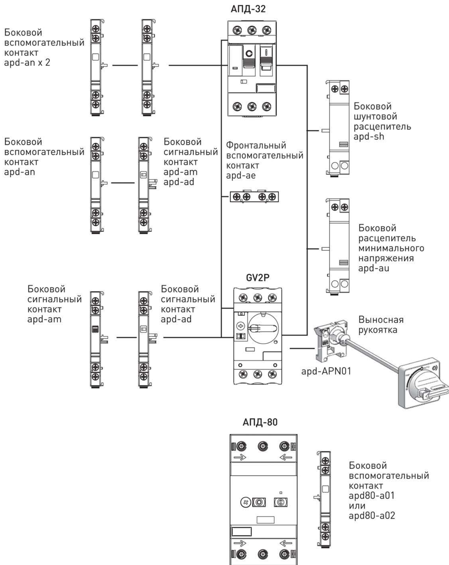
Рис. 1 – Схема установки дополнительных аксессуаров
