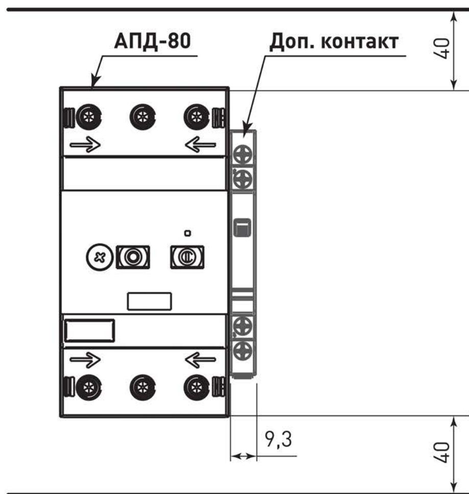
Рис. 11 – Габаритные размеры АПД-80
