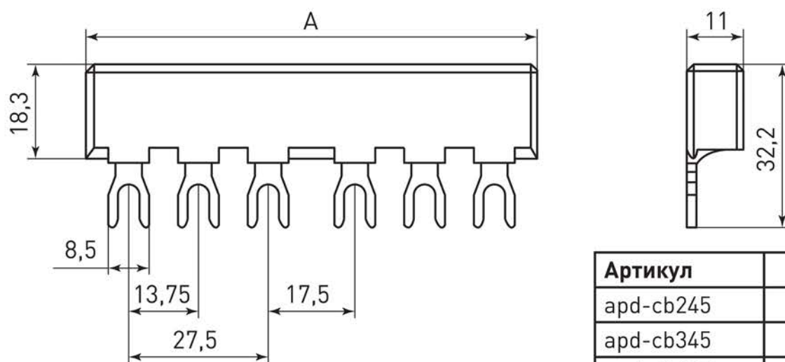
Рис. 6 – Габаритные размеры соединительного блока АПД/GV2 (Артикул: apd-cb)
