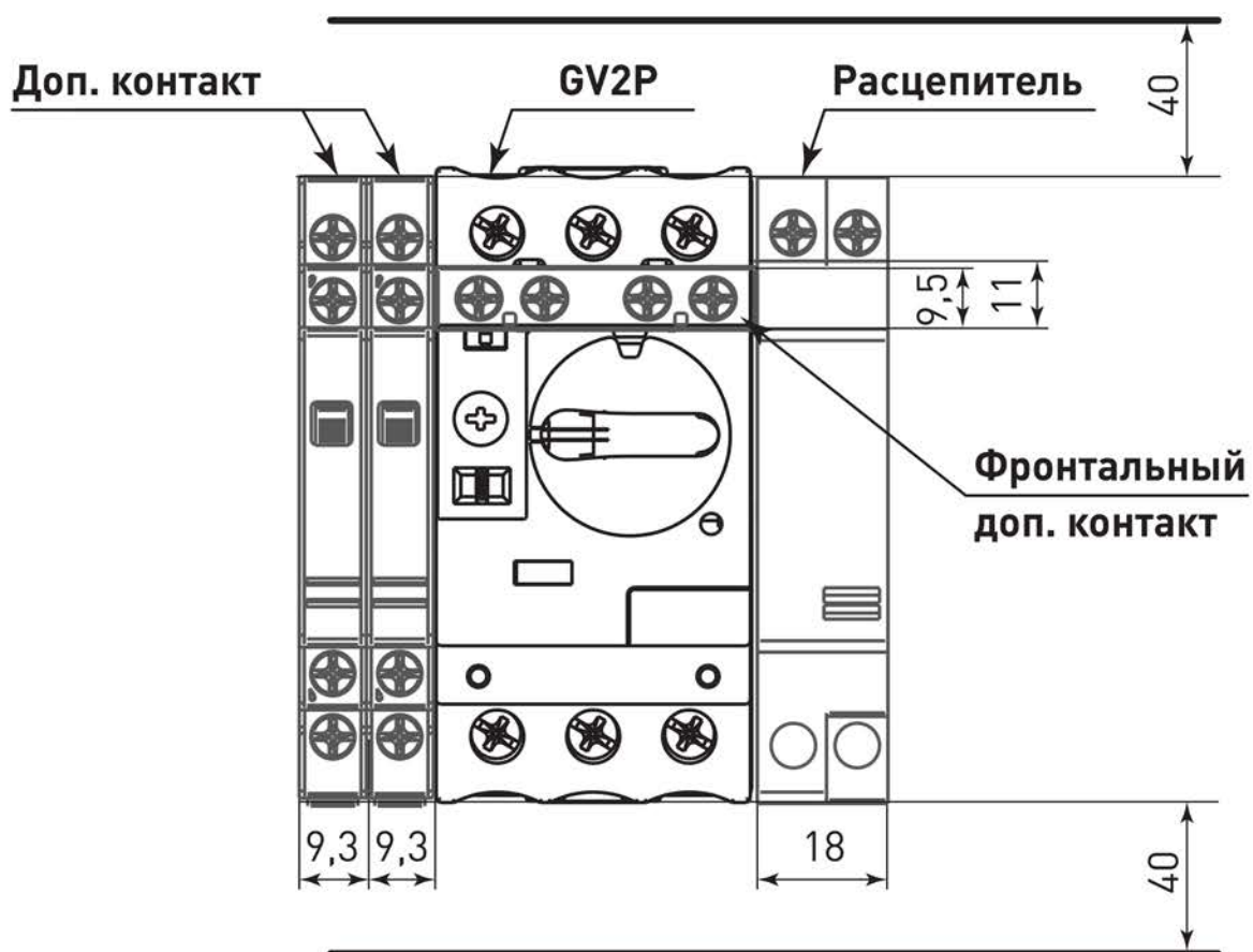
Рис. 10 – Габаритные размеры GV2P
