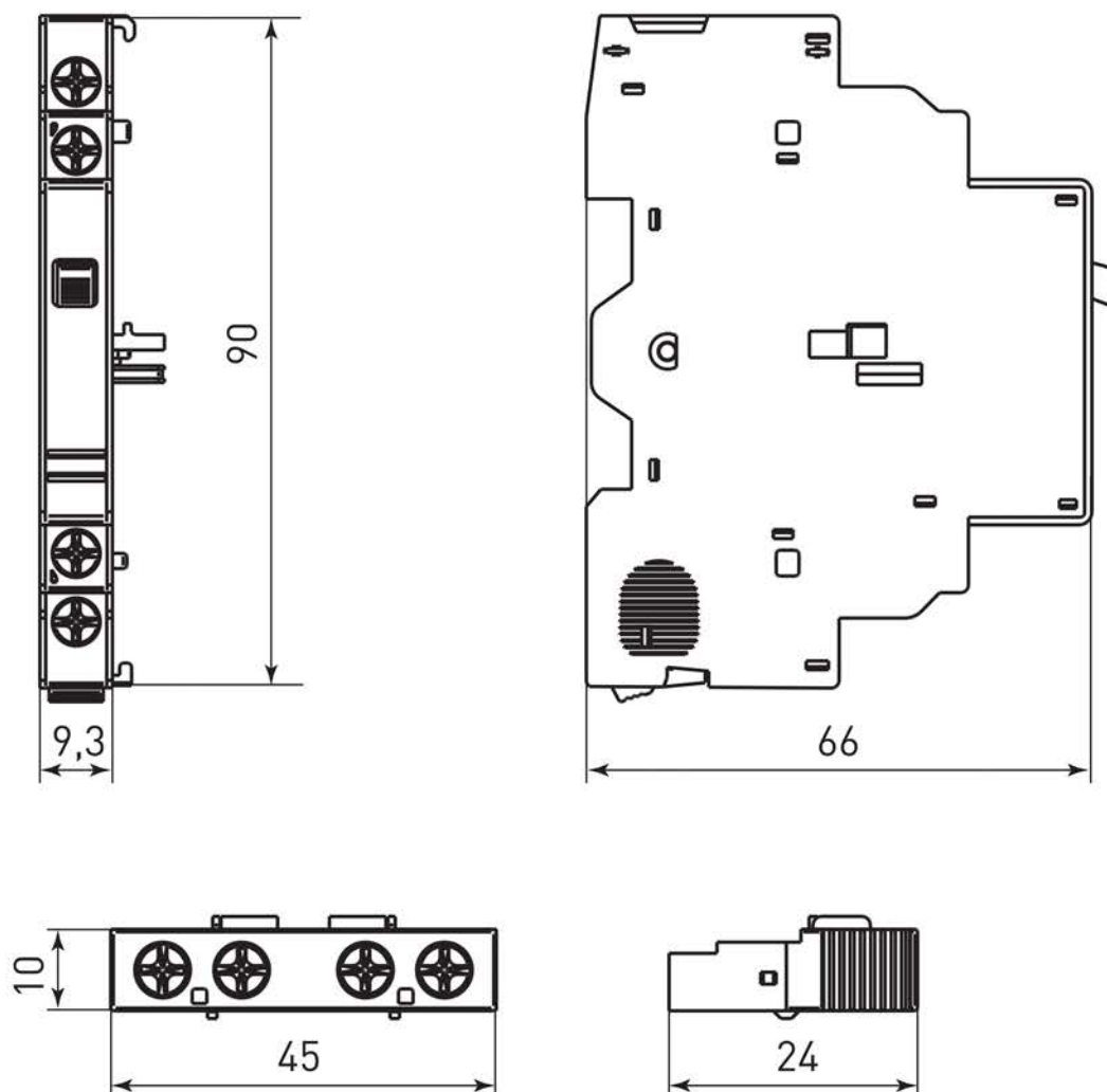
Рис. 4 – Габаритные размеры вспомогательных контактов
