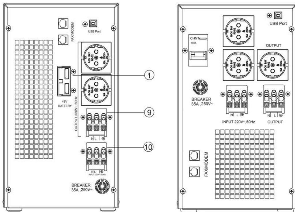
Рисунок 4 – Задняя панель ИБП ELT-5000VA-1-004-S, ELT-5000VA-1-L-S
