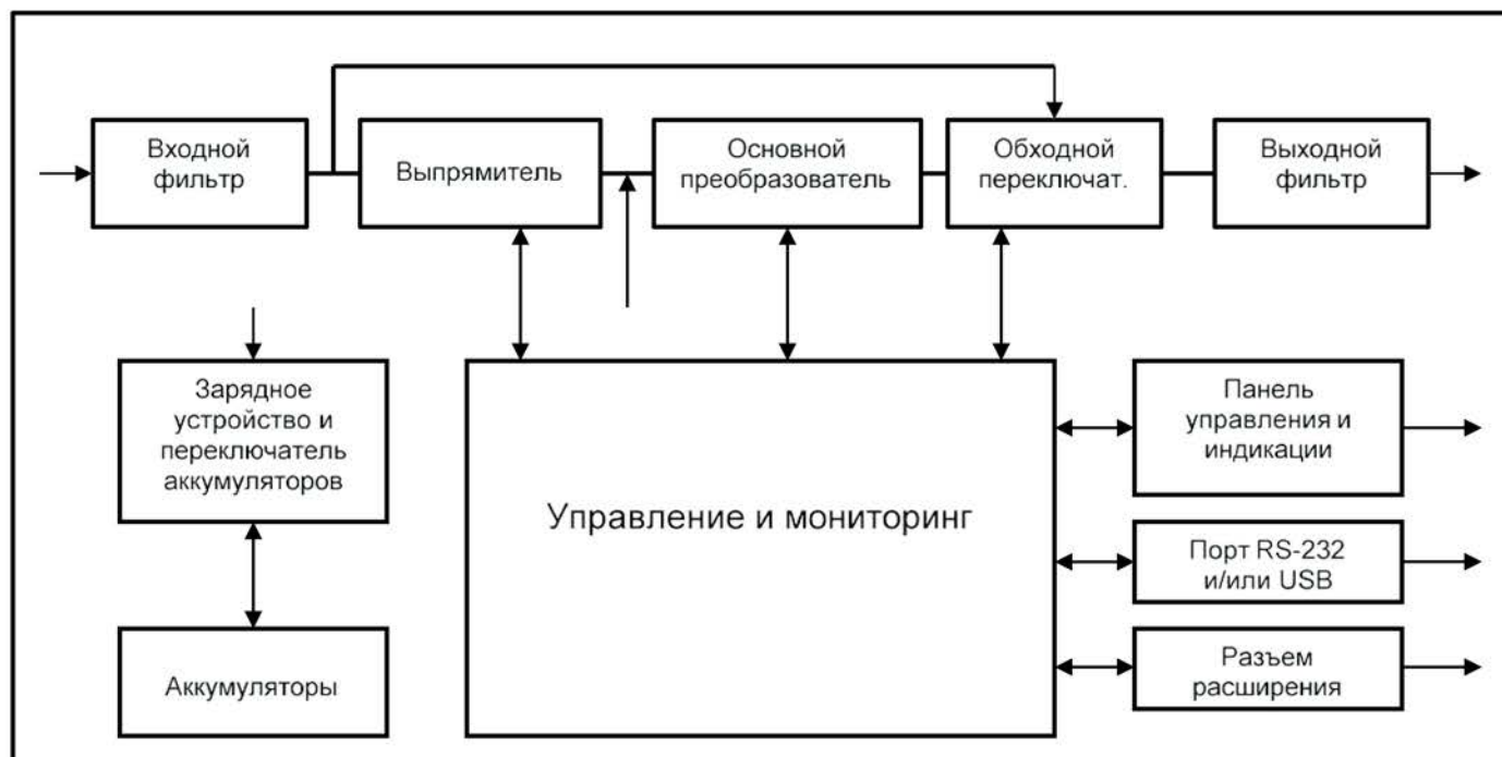
Рисунок 1 – Блок-схема ИБП
