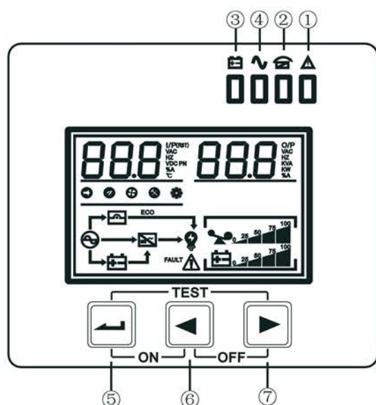
Рисунок 6 – Панель управления
