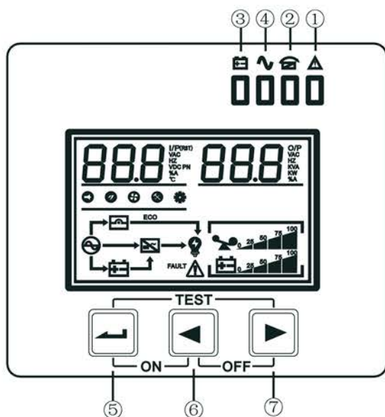
Рисунок 6 – Панель управления
