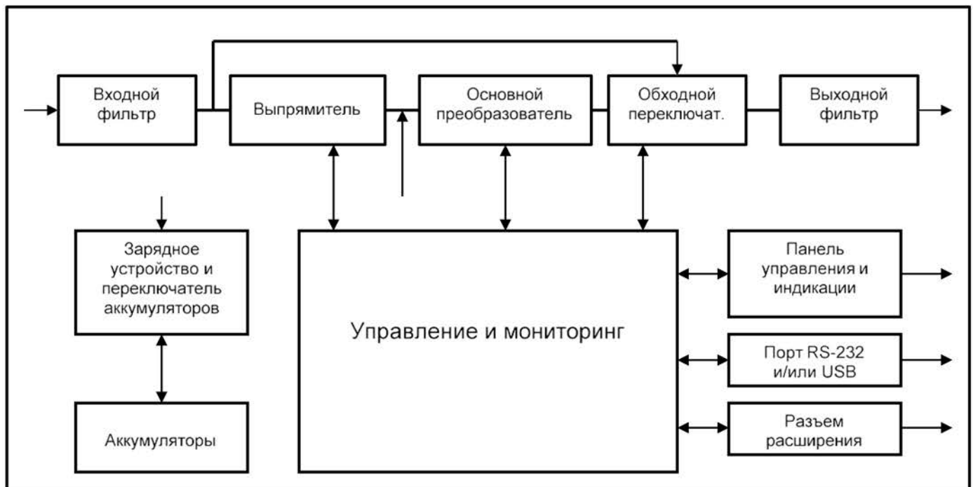
Рисунок 1 – Блок-схема ИБП
