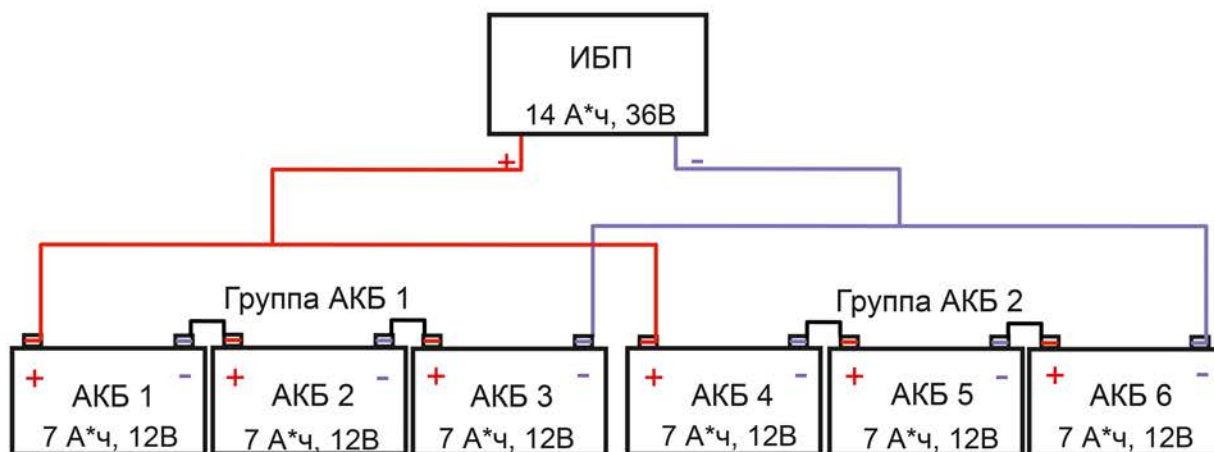
Рисунок 6 – Схема параллельно – последовательного подключения 6 АКБ батарейного кабинета.
