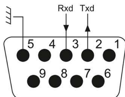
Рисунок 4 – Разъем RS-232
