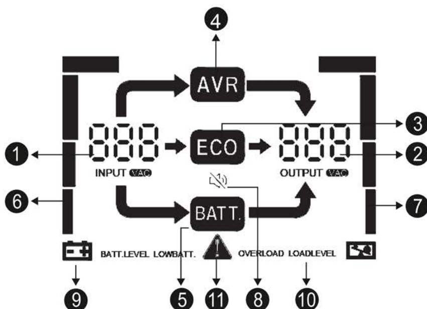
Рисунок 2 – Дисплей ИБП
