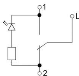
г) выключатель одноклавишный проходной с индикацией / pass- through 1-gang switch with indication / индикациясы бар бір пернелі өтпелі ажыратқыш / intrerupator singură de trecere prin cu indicatie / нэг даралттай нэвт гаралтай led гэрэлтэй унтраалга / indikatsiyali o'tuvchi bitta klavishli o'chirgich
