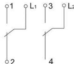
д) выключатель двухклавишный проходной / pass- through 2-gang switch / екі пернелі өтпелі ажыратқыш / intrerupator dublu de trecere prin / хоёр даралттай нэвт гаралтай унтраалга / indikatsiyali ikkita klavishli o'chirgich
