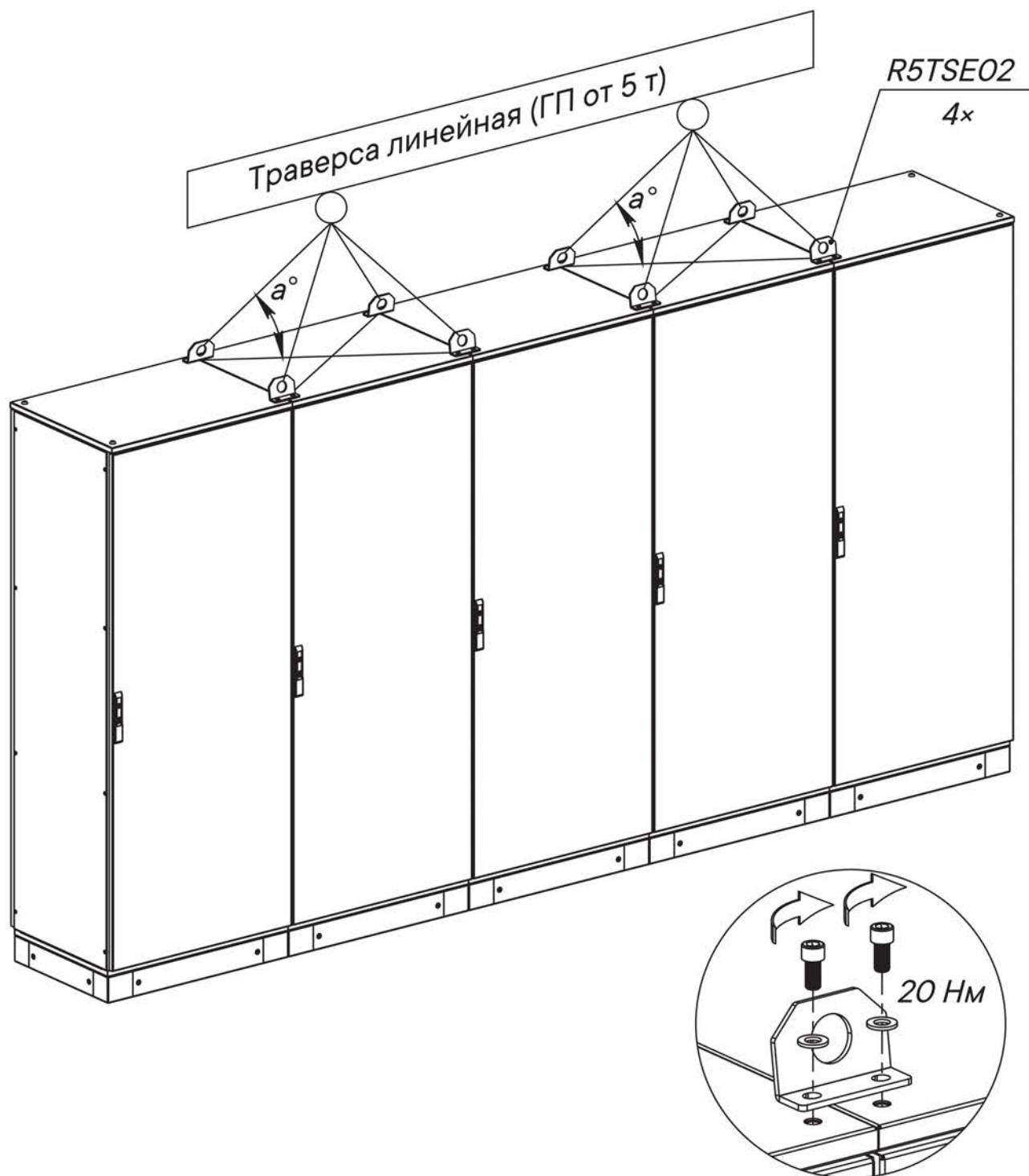
Схема распределения масс шкафов в сборке:
