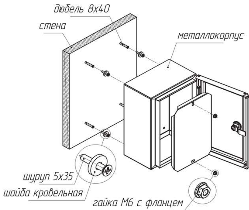
Рис. 1.1. Схема настенного монтажа
