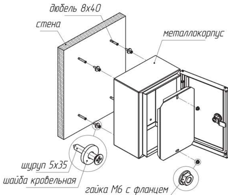
Рис. 1.1. Схема настенного монтажа.
