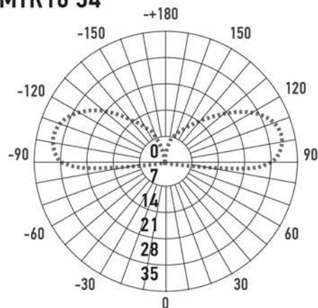
MTR16 34
